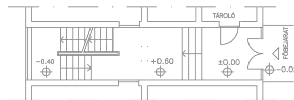
b./ ALÁPINCÉZETT, EMELT FÖLDSZINTI PADLÓVONAL
