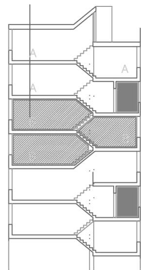
B./ OLDALFOLYOSÓS ELRENDEZÉS, FÉLSZINT-ELTOLÁSOS LAKÁSOKKAL
