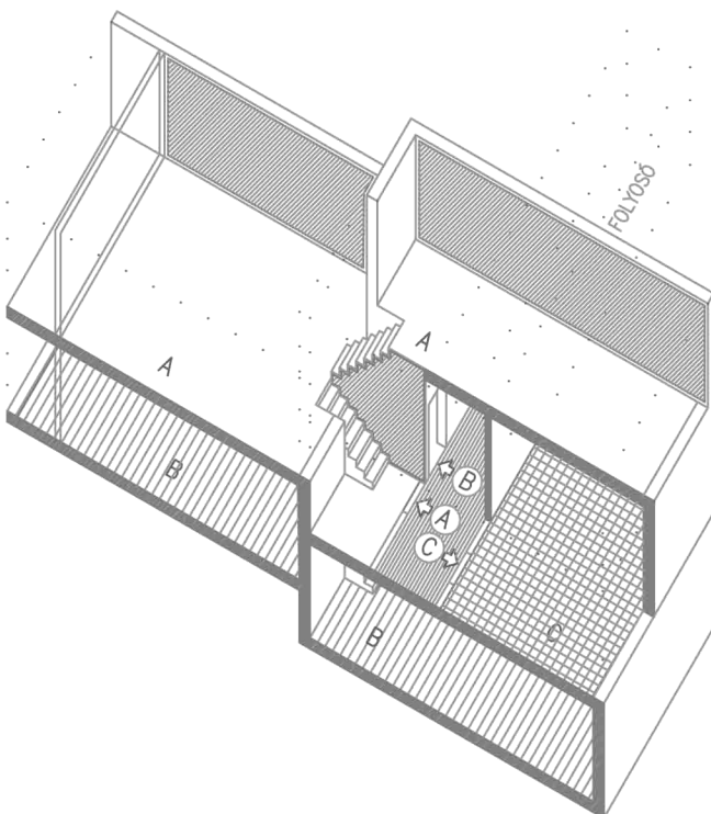
C./ BELSŐFOLYOSÓS ELRENDEZÉS FÉLSZINT-ELTOLÁSOS LAKÁSOKKAL
