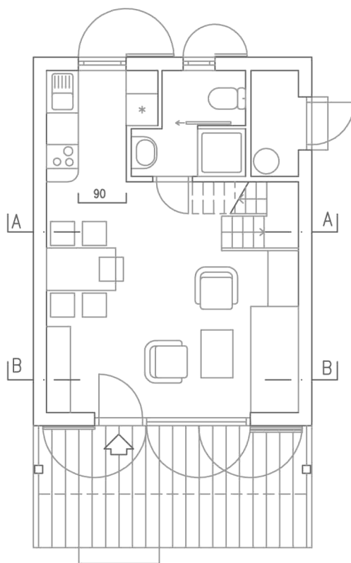
FÖLDSZINTI ALAPRAJZ
