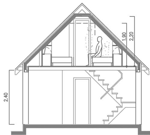
B-B METSZET
