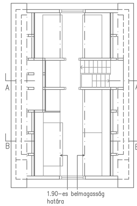
TETŐTÉRI ALAPRAJZ
