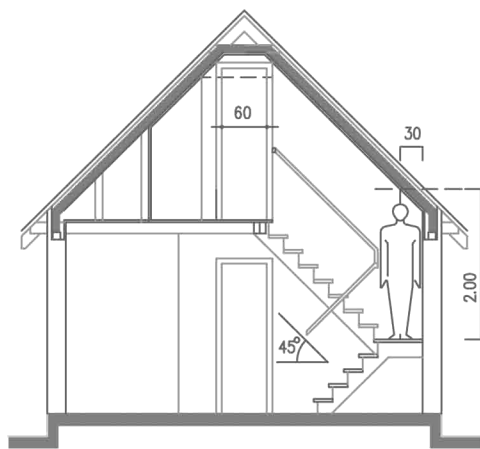
A-A METSZET
