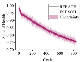
(f) DAE
