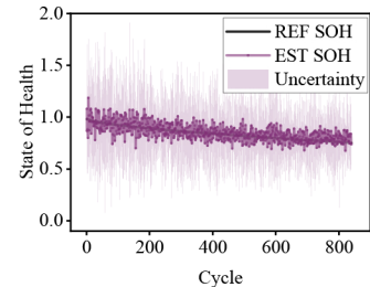
(e) DeNN
