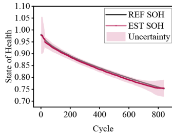
(g) SNGP
