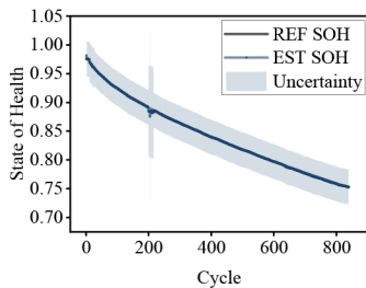
(b) GP-ICE
