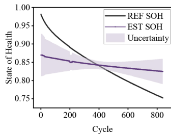
(d) SACN
