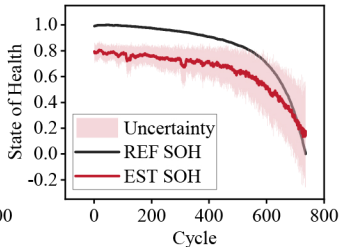
(d) Out-of-distribution SOH estimates
