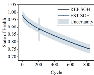
(b) GP-ICE
