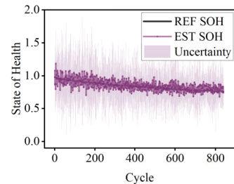
(e) DeNN
