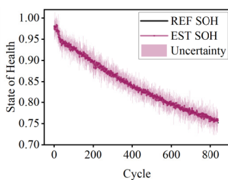
(f) DAE
