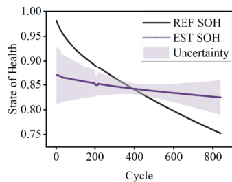
(d) SACN
