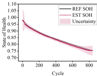
(g) SNGP
