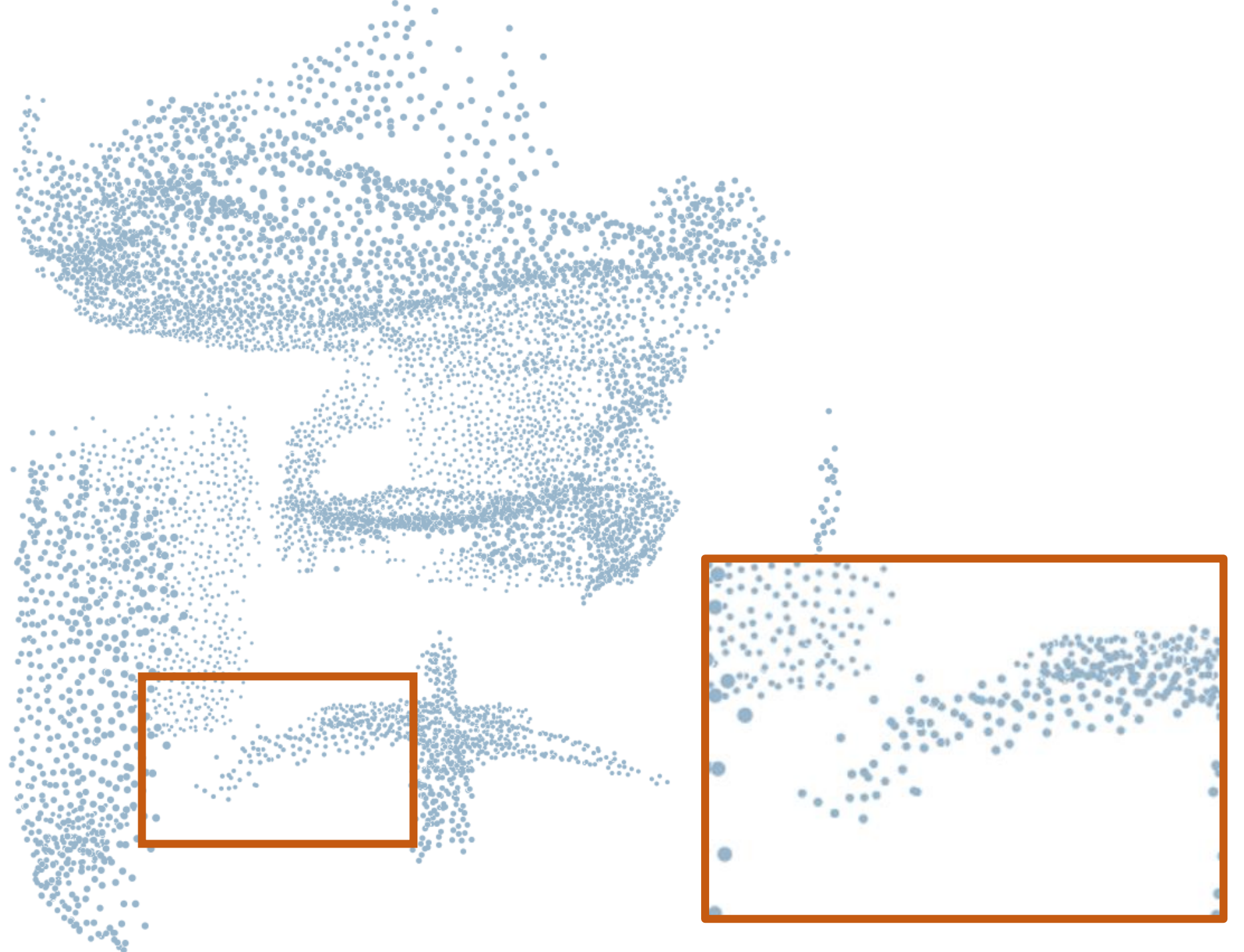
PU-GCN
