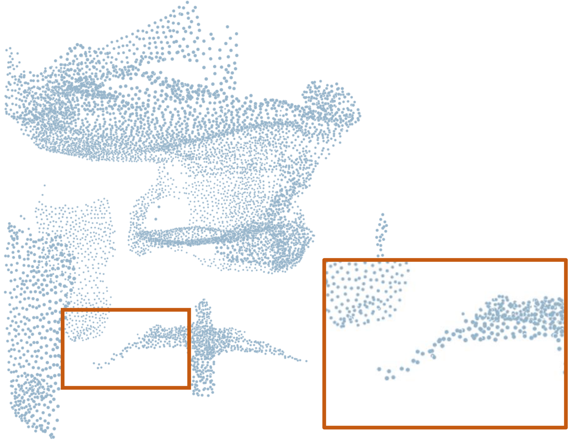
Dis-PU
