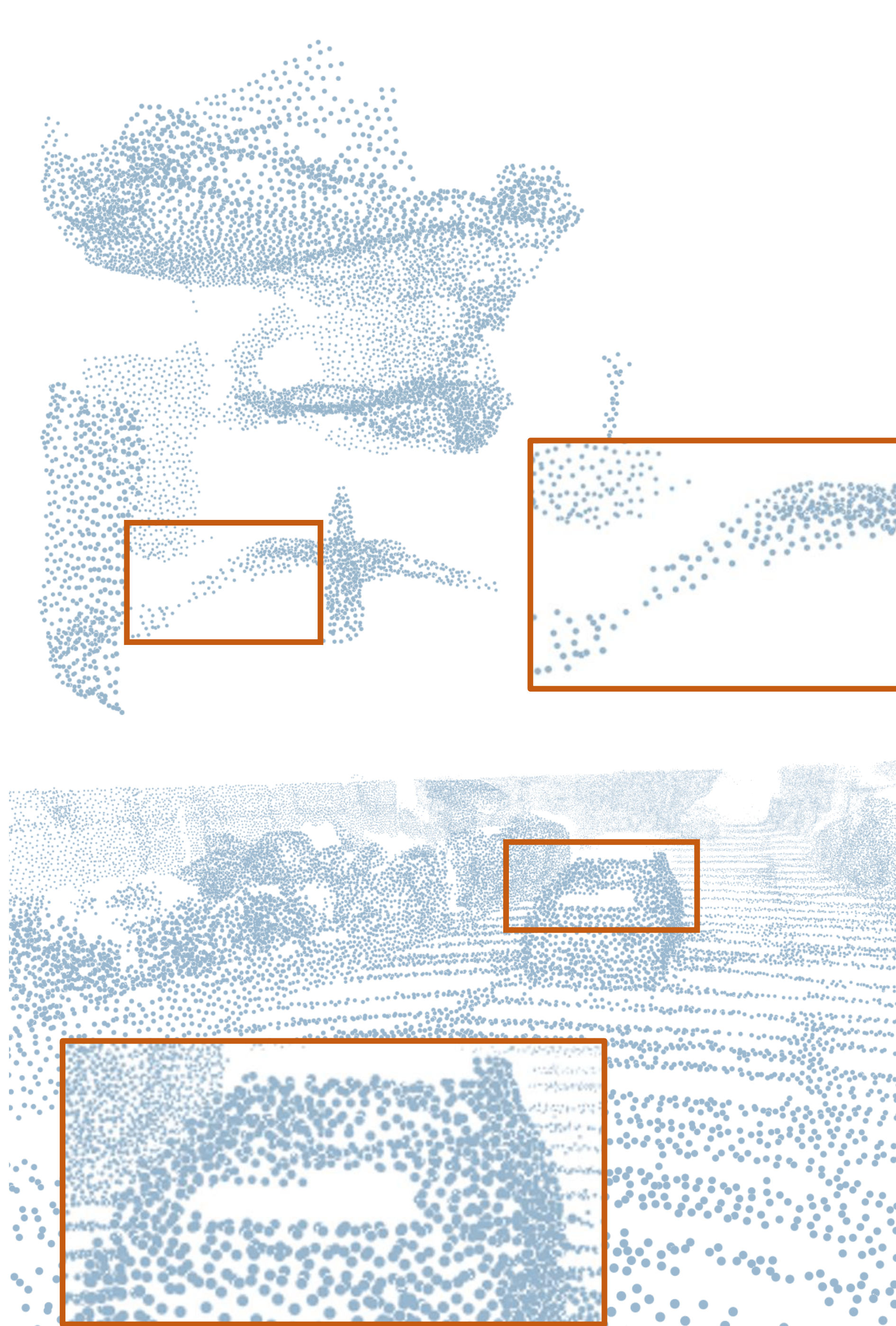
(b) PU-GAN
