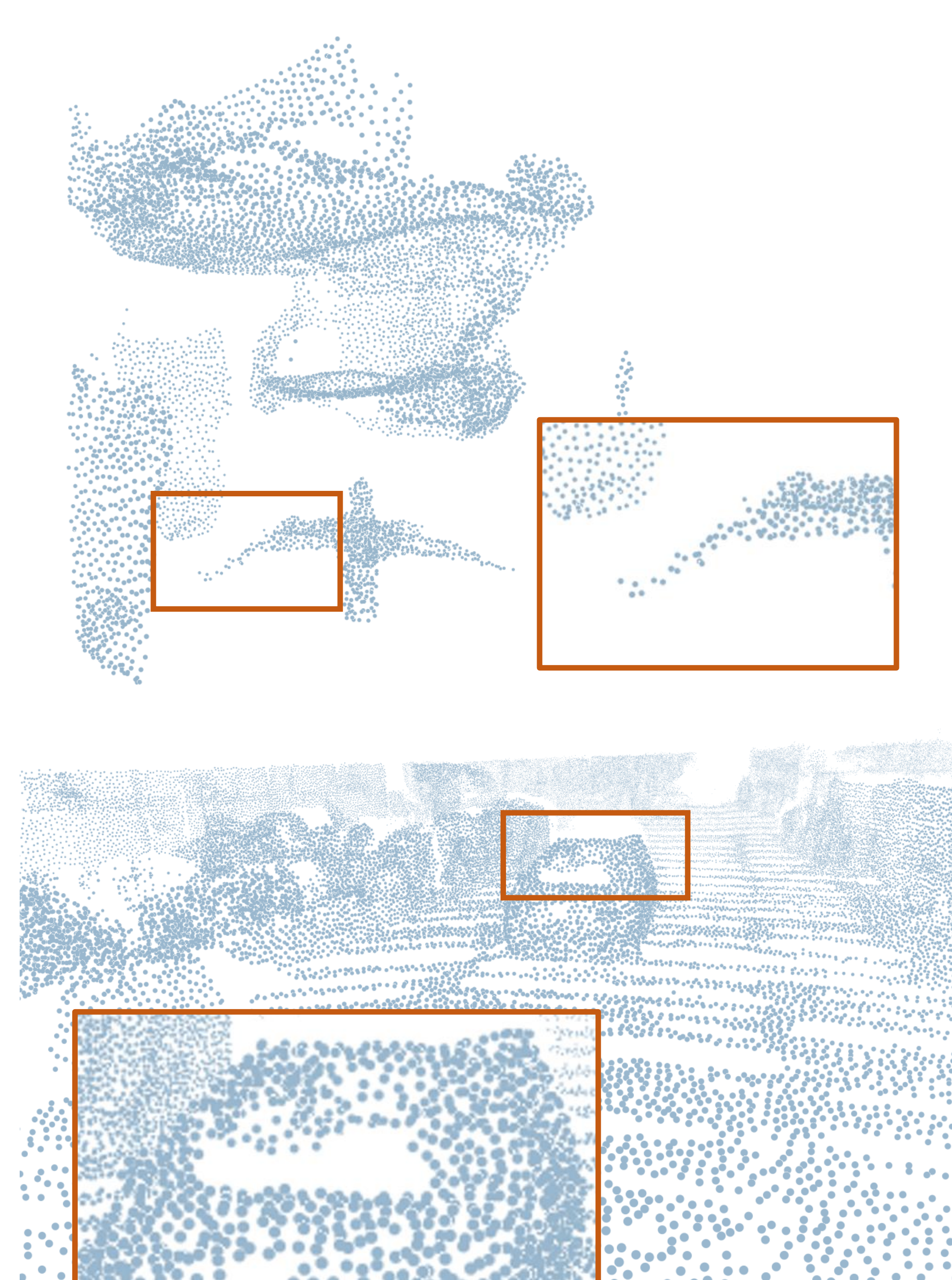
(d) Dis-PU
