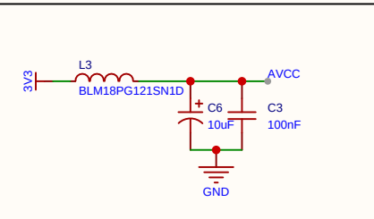
数模电压分离
