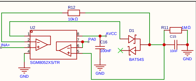
峰值检波电路
