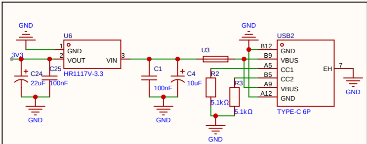
5V转3V3电源输入电路
