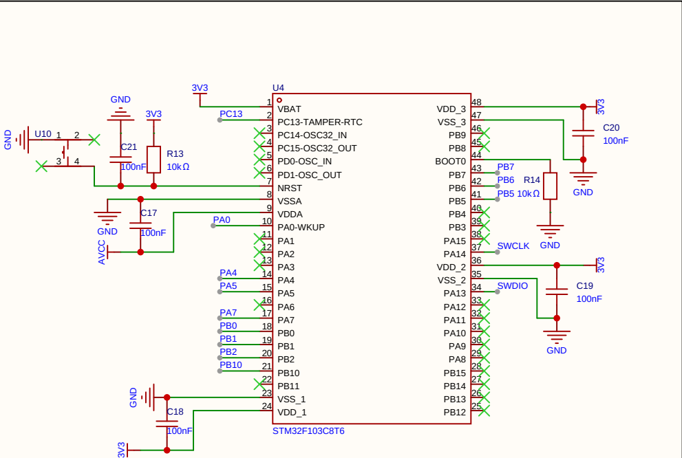
数模电压分离
