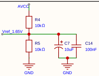
1.65V直流偏置基准
