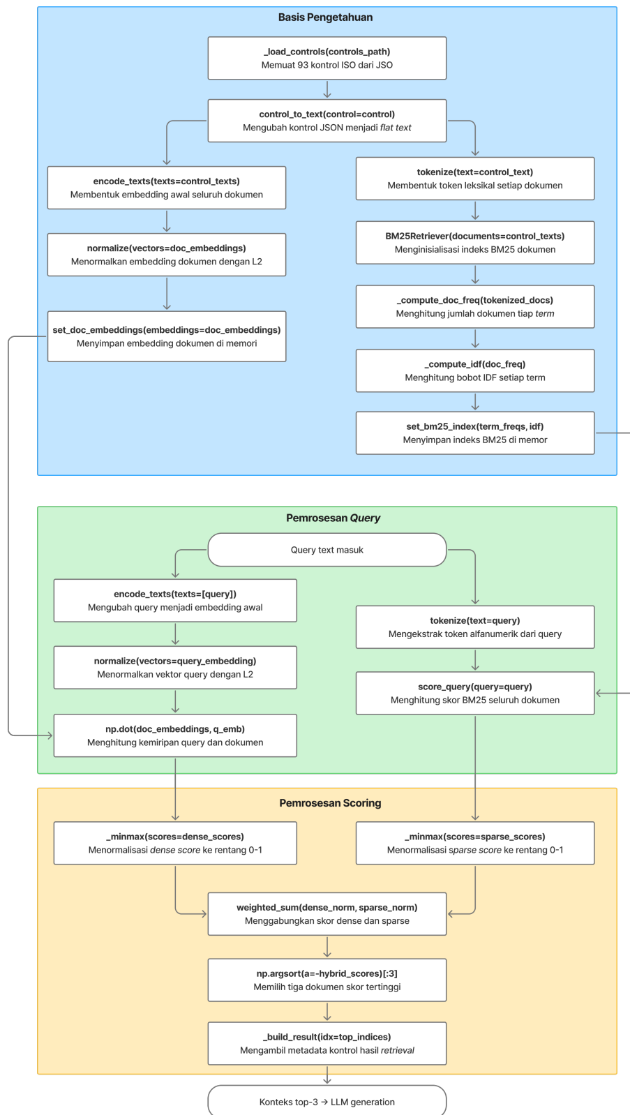
Gambar 3.6. Komponen hybrid retrieval pada sistem
