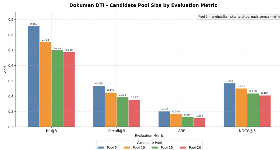
Gambar 4.27. Perbandingan metrik evaluasi berdasarkan ukuran candidate pool pada query dokumen DTI
