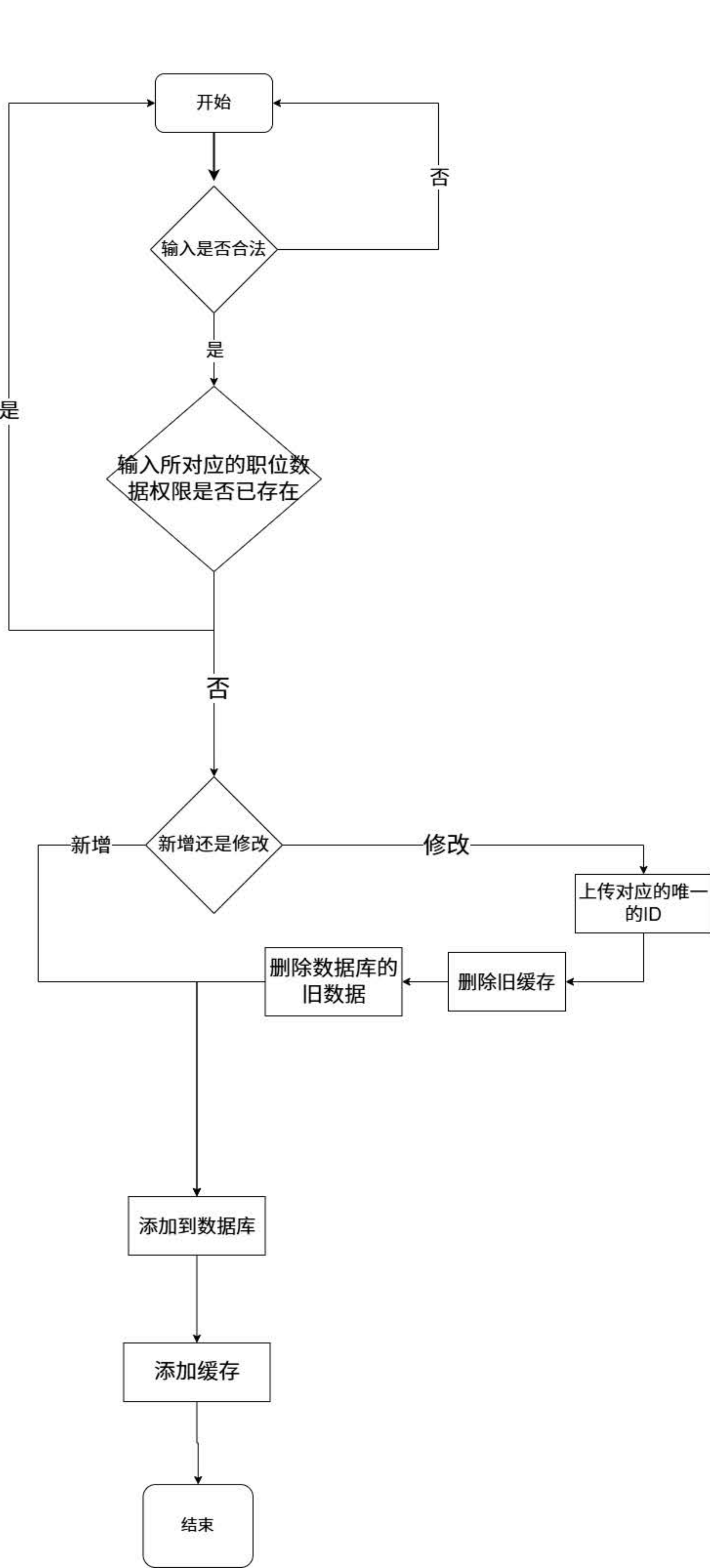
保存职位数据权限流程分析图
