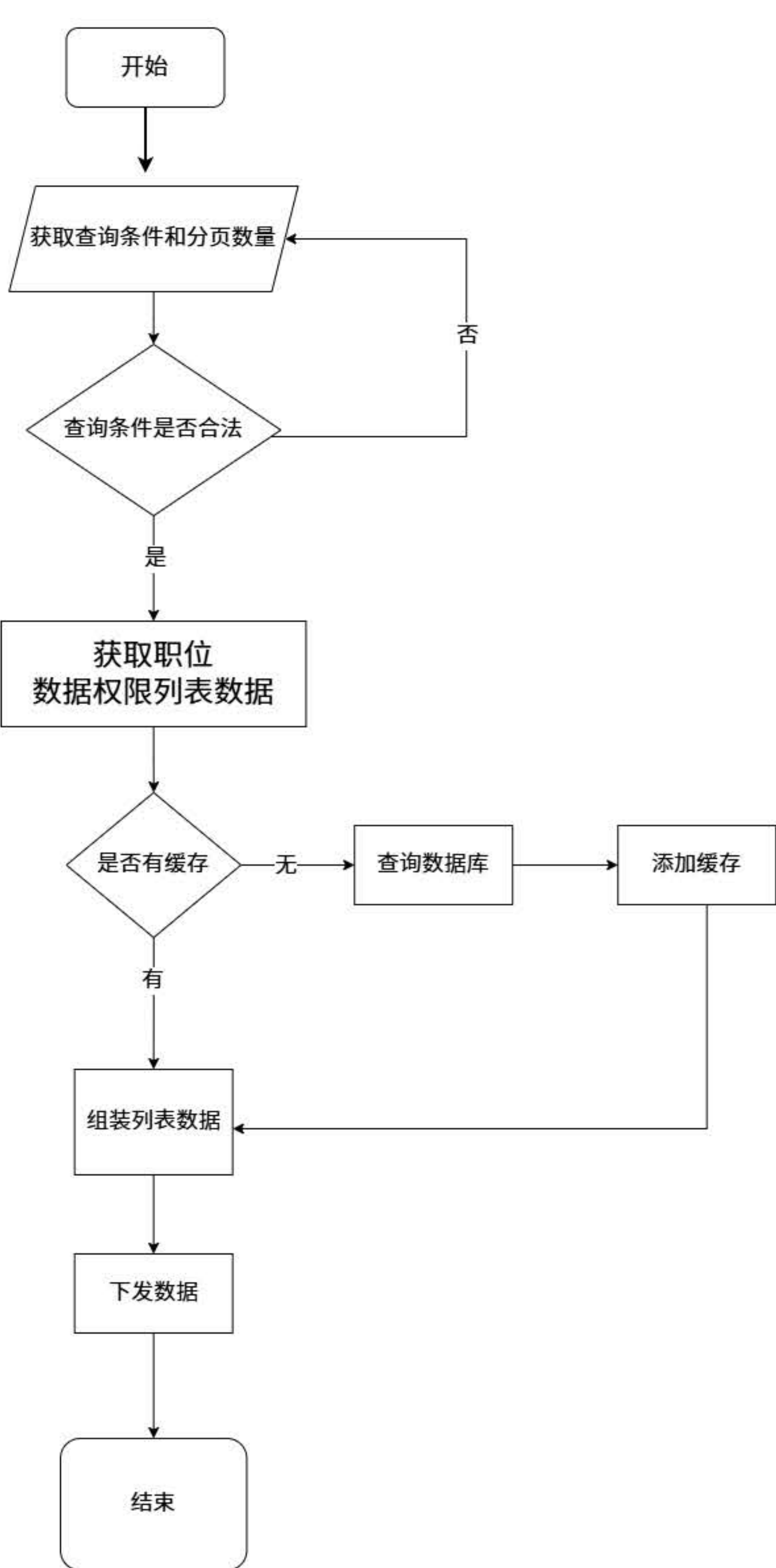
获取职位数据权限列表（条件+分页）流程分析图
