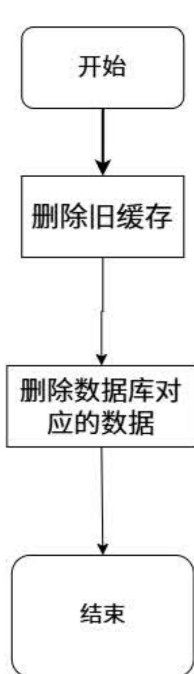
删除职位流程分析图
