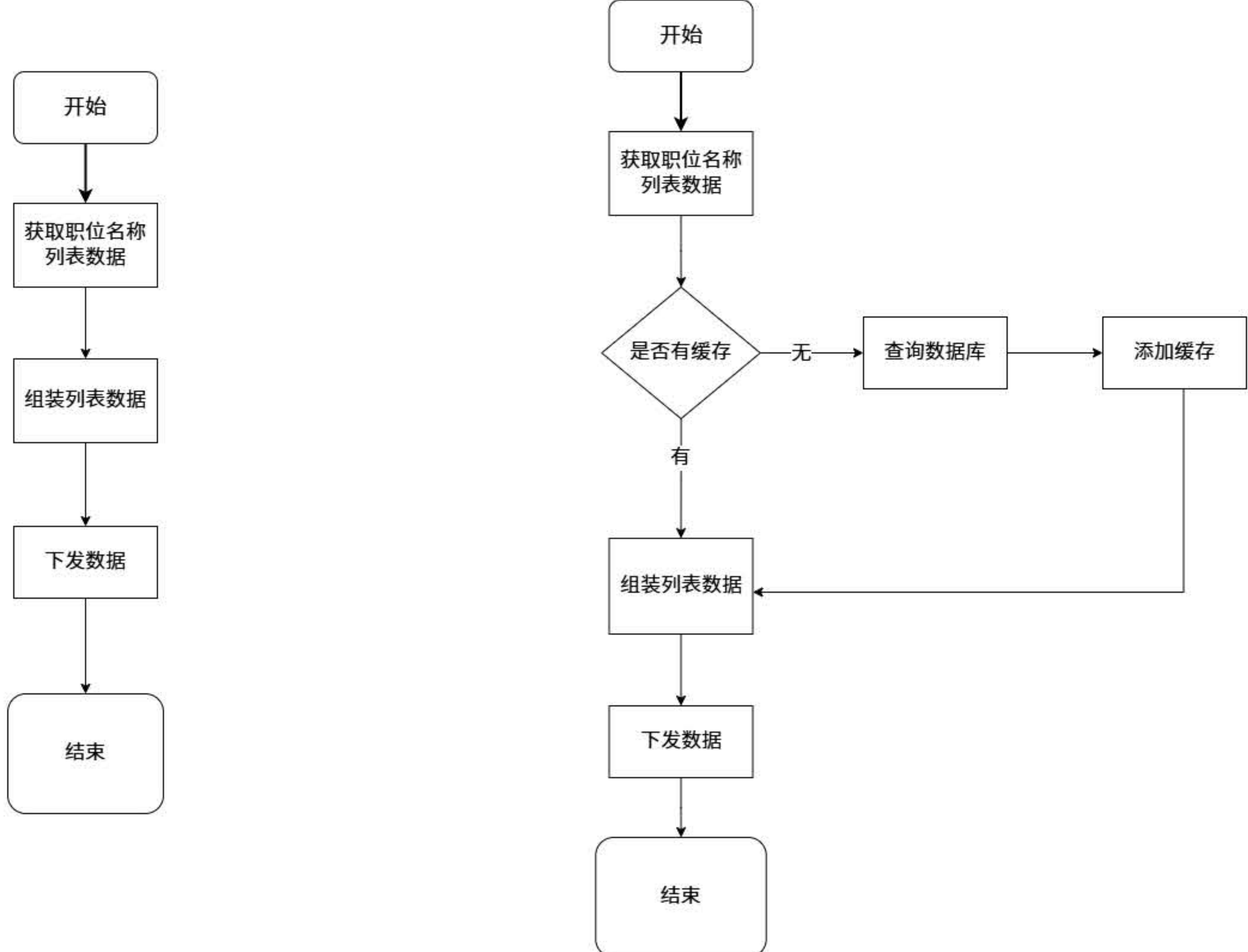
获取职位名称流程分析图
