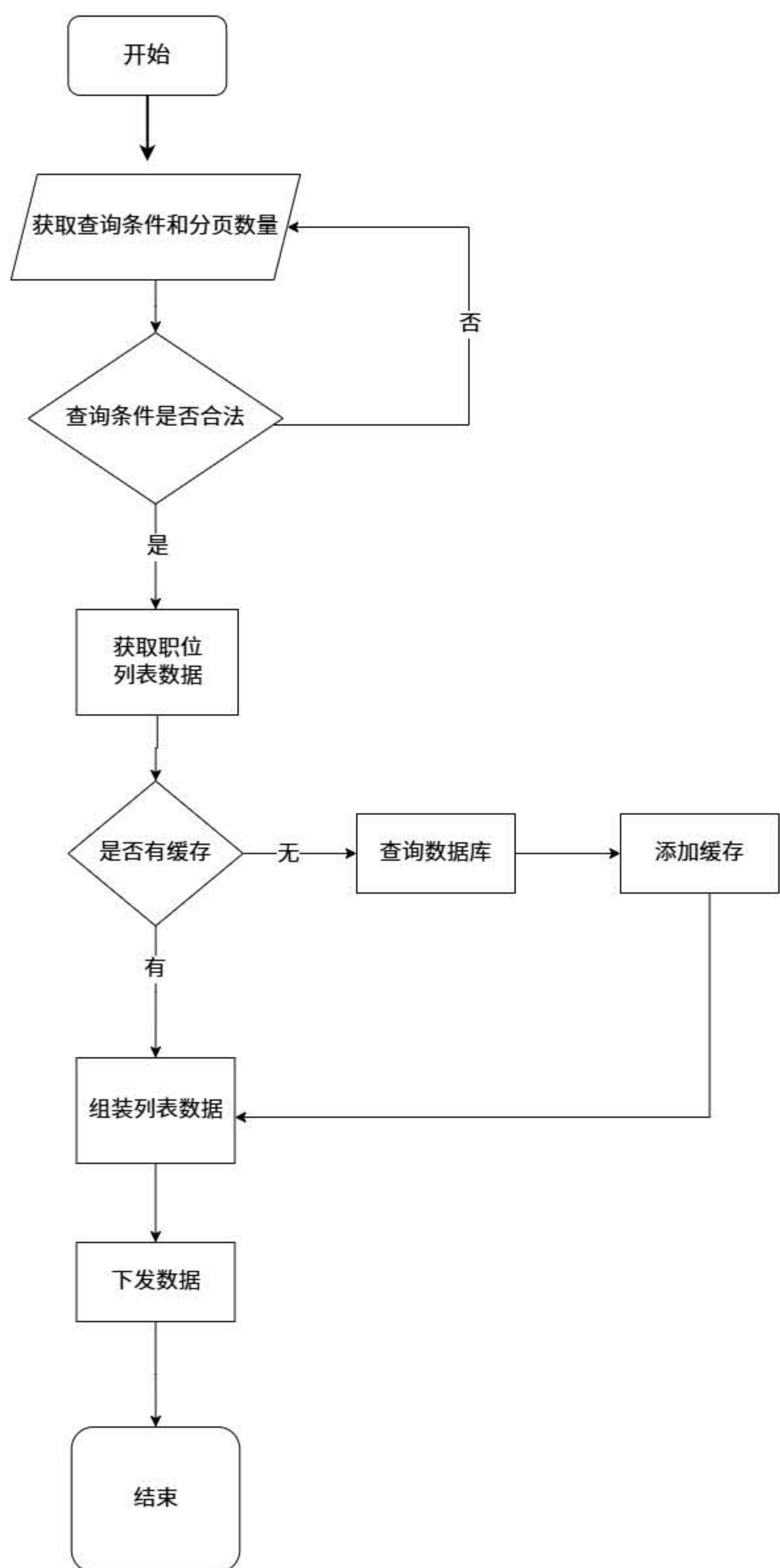
获取职位列表（条件+分页）流程分析图
