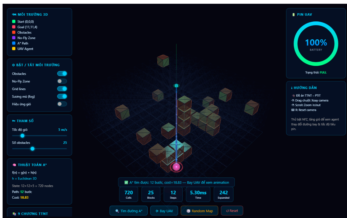
Hình 3. Demo 3D Three.js abstract - quỹ đạo UAV bay qua vùng có chướng ngại trên grid 12 \times 12 \times 5 .
