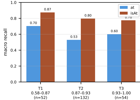
fr: macro-recall per OCR-quality tertile
