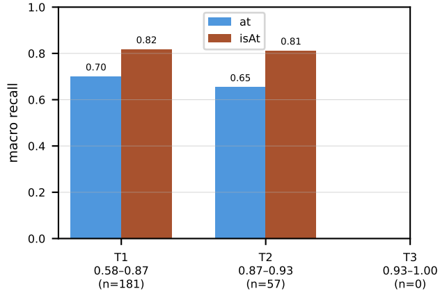
de: macro-recall per OCR-quality tertile
