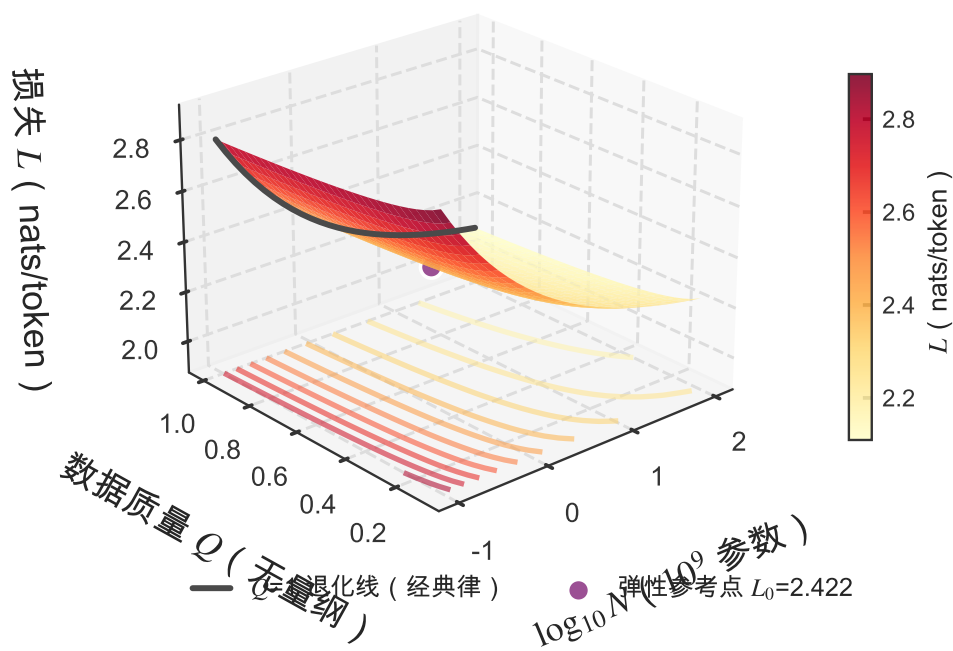
图 9 广义标度律损失曲面
