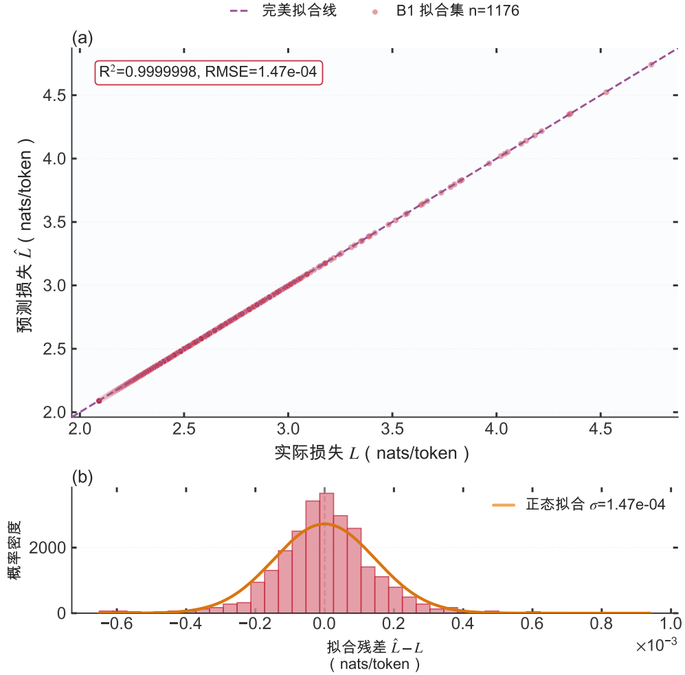
图 8 经典标度律拟合优度与残差
