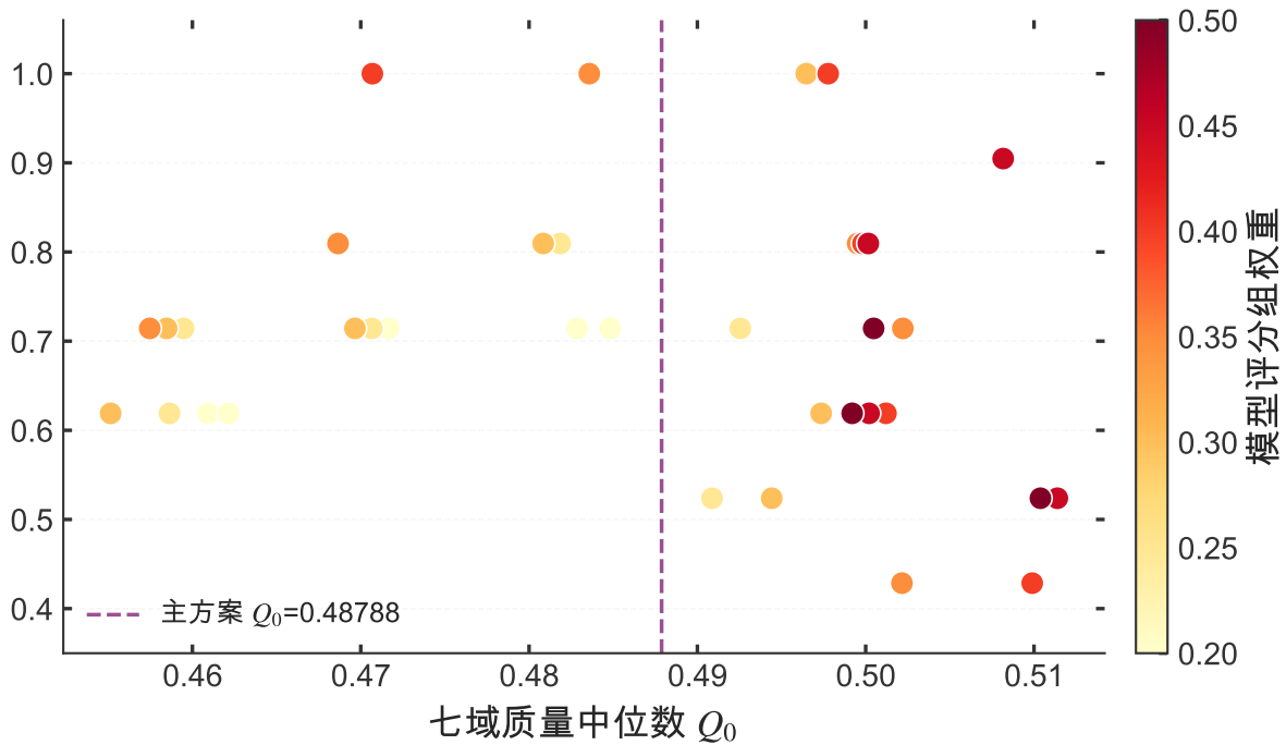
域序 Kendall 相关
