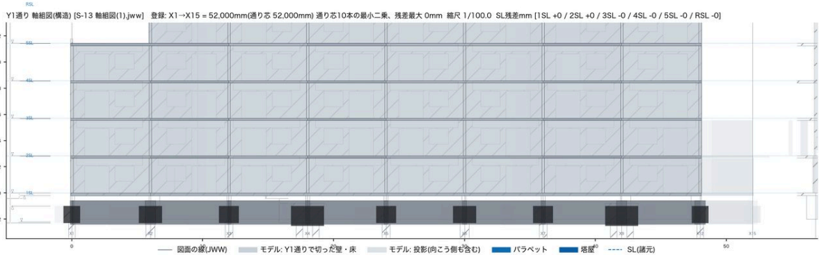
⑥ 通り断面: 上=構造 S-13 軸組図(1).jww Y1通り、下=意匠 立面図。登録は通り芯線と SL 線(文字位置ではない)
