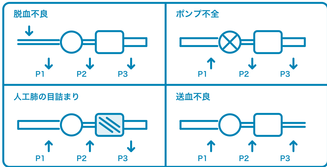
図8. 回路内圧の4象限（表29の図解）。各象限の下に矢印が P1・P2・P3 の動く向き。左上 脱血不良＝P1 が大きな陰圧へ振れ、P2・P3 も下がる（P1 だけが際立って落ちるのが決め手）。右上 ポンプ不全＝P1 が上がり、P2・P3 がともに下がる。左下 人工肺の目詰まり＝P2 が上がり P3 が下がる（P2-P3 が開く）。右下 送血不良＝P2 も P3 も上がる（P2-P3 は開かない）。流量はいずれも低下する。
