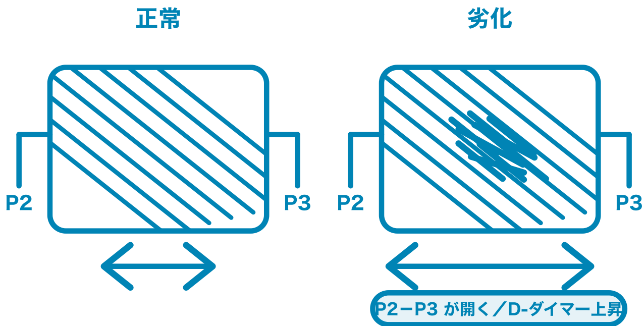
図10. 人工肺の劣化と P2-P3。左（正常）＝中空糸が均一で、人工肺の入口（P2）と出口（P3）の圧較差は小さい（下の両矢印が短い）。右（劣化）＝フィブリン沈着で中空糸が目詰まりし、P2-P3 が開く（両矢印が長い）。手がかりは P2-P3 > 50 \text{ mmHg} / 送血側 \text{SaO}_2 < 98\% / D-ダイマー上昇。 定期的な回路交換は行わないが 、この所見が揃えば交換を考慮する（表29・表31）。
