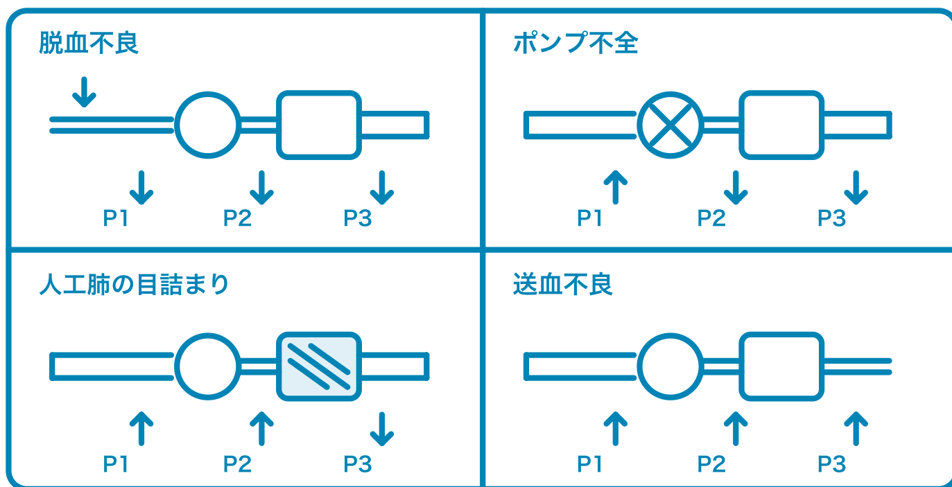
図11. 回路内圧の4象限（表38の図解）。各象限の下に矢印がP1・P2・P3の動く向き。左上 脱血不良＝P1が大きな陰圧へ振れ、P2・P3も下がる（P1だけが際立って落ちるのが決め手）。右上 ポンプ不全＝P1が上がり、P2・P3がともに下がる。左下 人工肺の目詰まり＝P2が上がりP3が下がる（P2-P3が開く）。右下 送血不良＝P2もP3も上がる（P2-P3は開かない）。流量はいずれも低下する。
