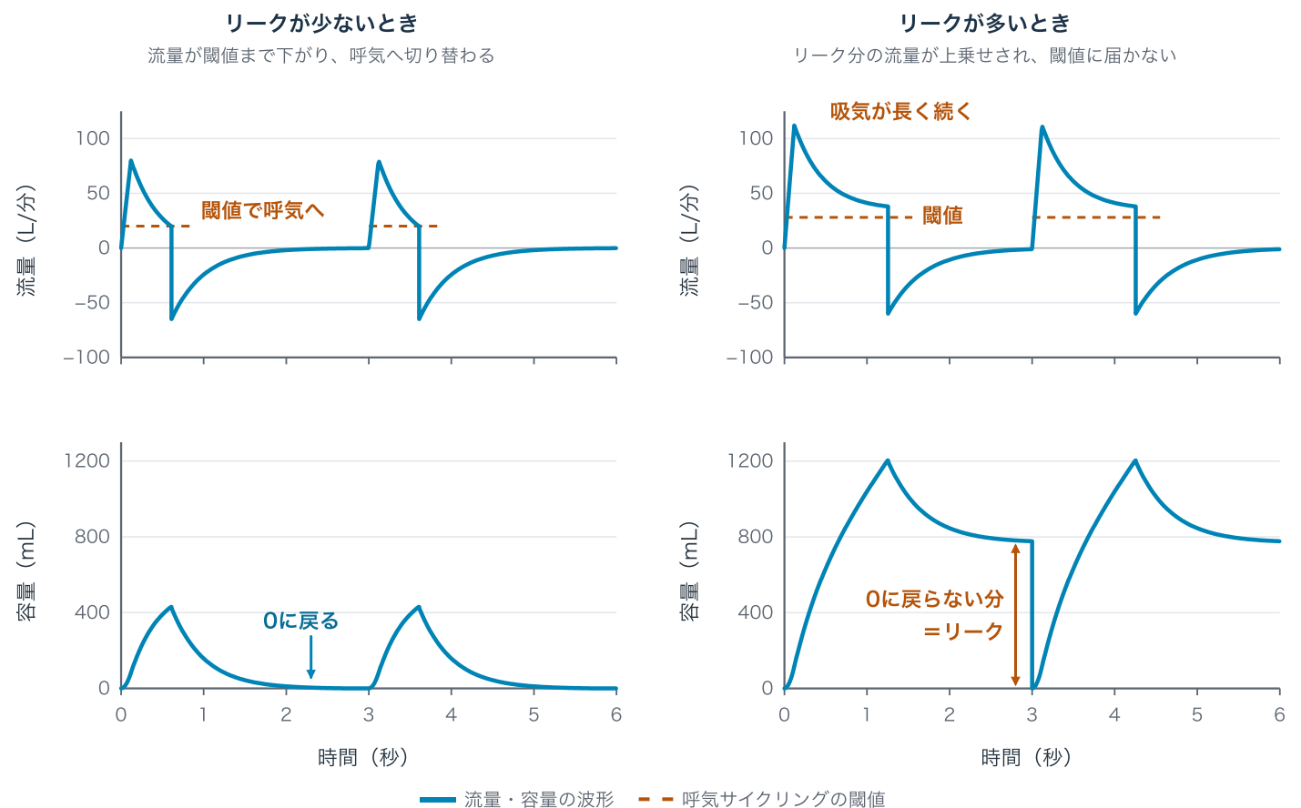
図7. リークが少ないときと多いときの流量と容量の波形（模式図）。
