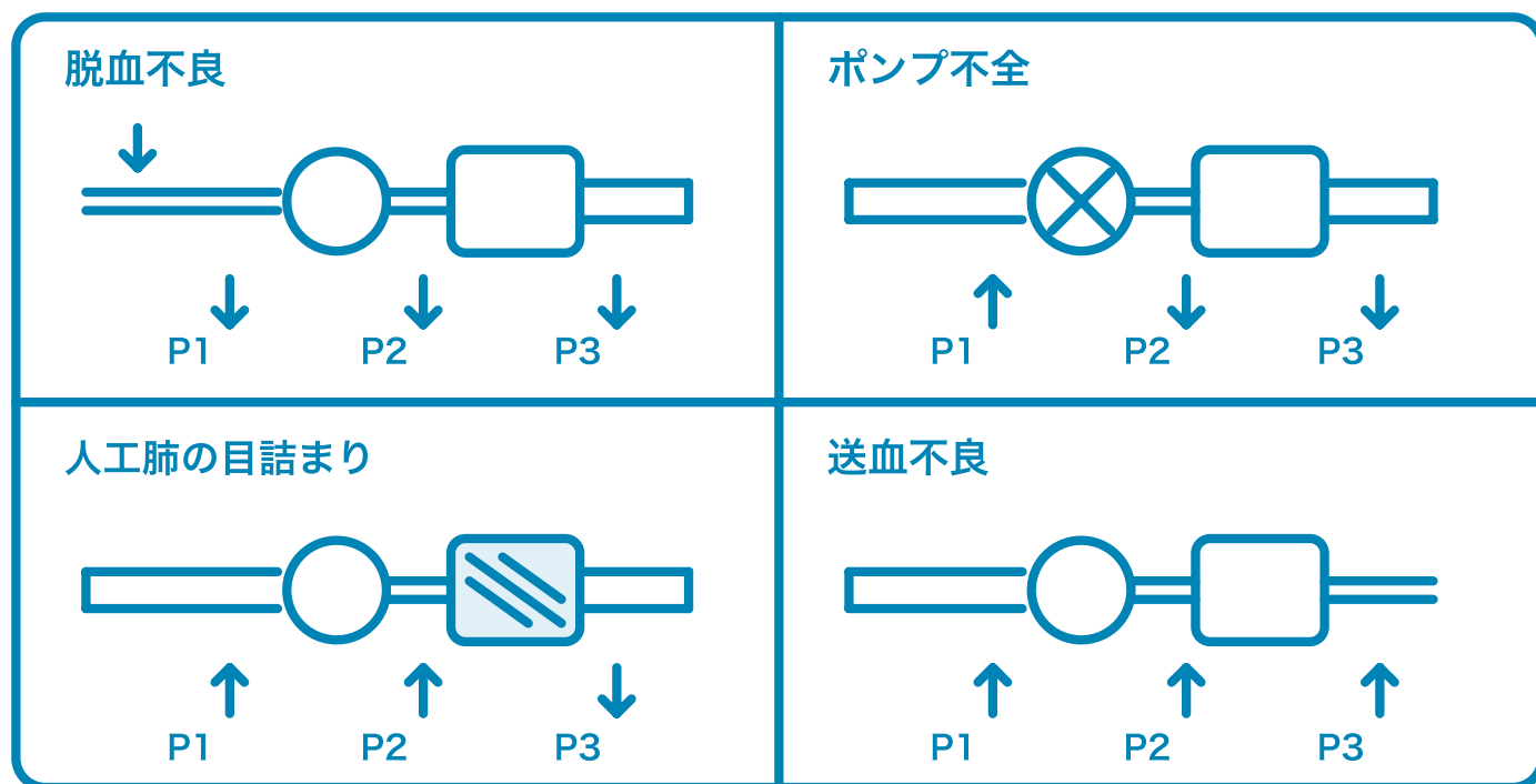
図7. 回路内圧の4象限（表27 の図解）。各象限の下矢印が P1・P2・P3 の動く向き。左上 脱血不良=P1 が大きな陰圧へ振れ、P2・P3 も下がる（P1 だけが際立って落ちるのが決め手）。右上 ポンプ不全=P1 が上がり、P2・P3 がともに下がる。左下 人工肺の目詰まり=P2 が上がり P3 が下がる（P2-P3 が開く）。右下 送血不良=P2 も P3 も上がる（P2-P3 は開かない）。流量はいずれも低下する。
