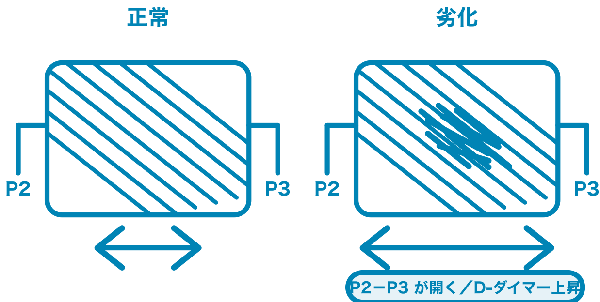
図14. 人工肺の劣化と P2-P3。左（正常）＝中空系が均一で、人工肺の入口（P2）と出口（P3）の圧較差は小さい（下の両矢印が短い）。右（劣化）＝フィブリン沈着で中空系が目詰まりし、P2-P3 が開く（両矢印が長い）。手がかりは P2-P3 > 50 mmHg / 送血側 SaO 2 < 98% / D-ダイマー上昇。定期的な回路交換は行わないが、この所見が揃えば交換を考慮する（表39・表41）。
