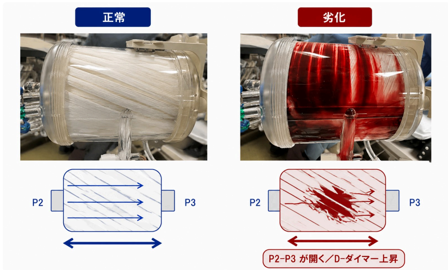
図15. 人工肺の劣化と P2-P3。左＝正常（中空糸が均一、圧較差は小さい）、右＝劣化（フィブリン沈着で目詰まりし、P2-P3 が開く）。
