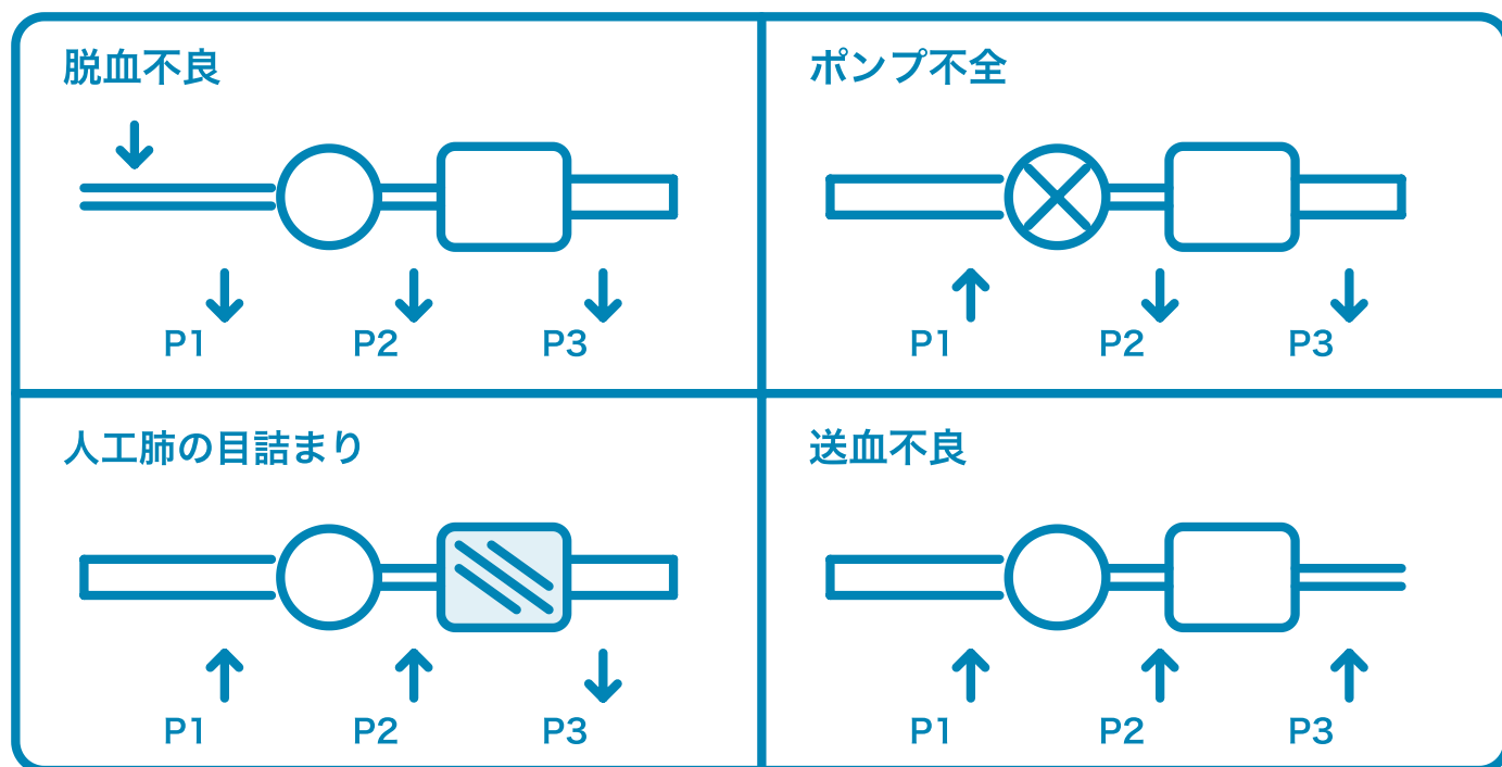
図7. 回路内圧の4象限（表31 の図解）。各象限の下矢印が P1・P2・P3 の動く向き。 左上 脱血不良 =P1 が大きな陰圧へ振れ、P2・P3 も下がる（P1 だけが際立って落ちるのが決め手）。 右上 ポンプ不全 =P1 が上がり、P2・P3 がともに下がる。左下 人工肺の目詰まり =P2 が上がり P3 が下がる（P2-P3 が開く）。右下 送血不良 =P2 も P3 も上がる（P2-P3 は開かない）。流量はいずれも低下する。
