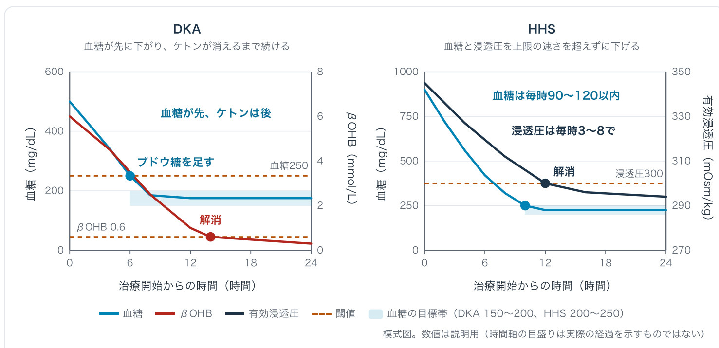
図5. 治療中の血糖・β OHB・浸透圧の経過 — DKAとHHSの対比。
