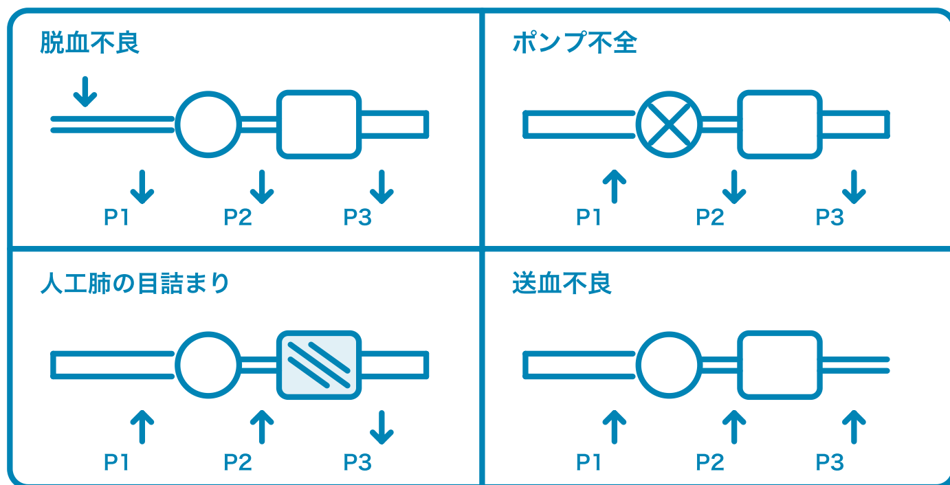
図7. 回路内圧の4象限（表30 の図解）。各象限の下矢印が P1・P2・P3 の動く向き。 左上 脱血不良 =P1 が大きな陰圧へ振れ、P2・P3 も下がる（P1 だけが際立って落ちるのが決め手）。 右上 ポンプ不全 =P1 が上がり、P2・P3 がともに下がる。左下 人工肺の目詰まり =P2 が上がり P3 が下がる（P2-P3 が開く）。右下 送血不良 =P2 も P3 も上がる（P2-P3 は開かない）。流量はいずれも低下する。
