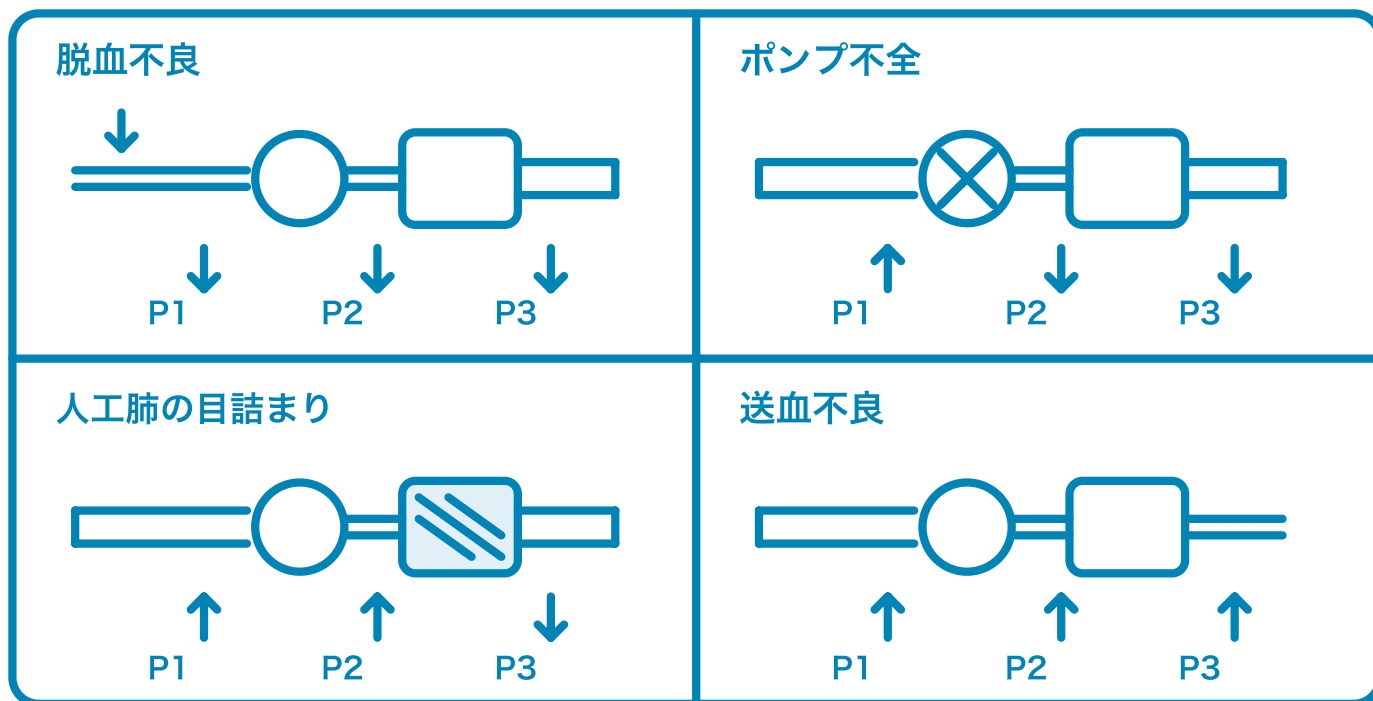
図12. 回路内圧の4象限（表40の図解）。各象限の下の矢印が P1・P2・P3 の動く向き。流量はいずれも低下する。
