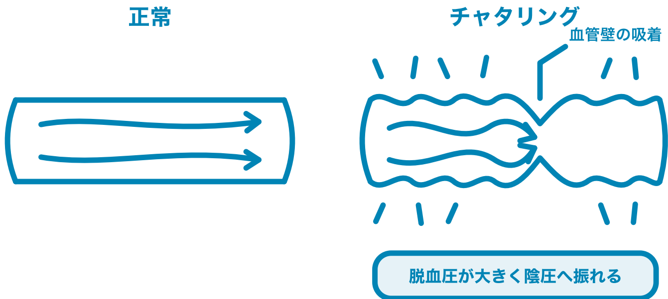
図13. チャタリング。左（正常）＝脱血管は安定し、血流も滑らか。右（チャタリング）＝血管壁が脱血管に吸着し、回路全体が細かく振動して血流が途切れる。このとき脱血圧は大きく陰圧へ振れる。最初の一手はモーター回転数を速やかに下げること、輸液や体位はその後（表40）。
