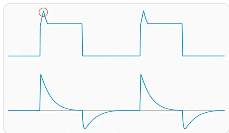
図10. NIVで見る6つの非同調の波形。
