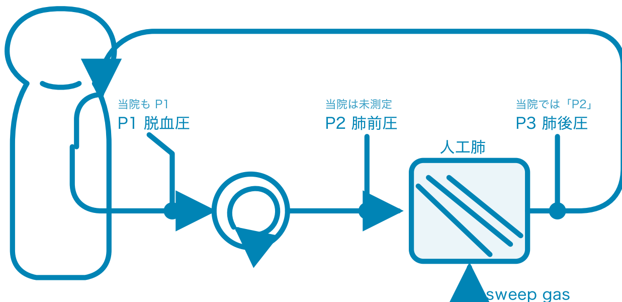
図1. VV-ECMO 回路の全体像と圧の測定点。患者から脱血した血液が遠心ポンプで送られ、人工肺でガス交換されて患者に戻る。P1=脱血圧 (ポンプ前・陰圧) / P2=肺前圧 (ポンプ後・人工肺前) / P3=肺後圧 (人工肺後)。sweep gas は人工肺の気相側に入る。基準値 (P1 > -120 (当院の運用閾値は -100) / P2 < 300 / P2-P3 < 50 mmHg) は §7-1。当院はこの3点のうち P1 と P3 の2点しか測っていない ——モニタの「P2」表示は図の P3 (肺後圧) で、 肺前圧を測っていないため P2-P3 は算出できない (§7-1)。
