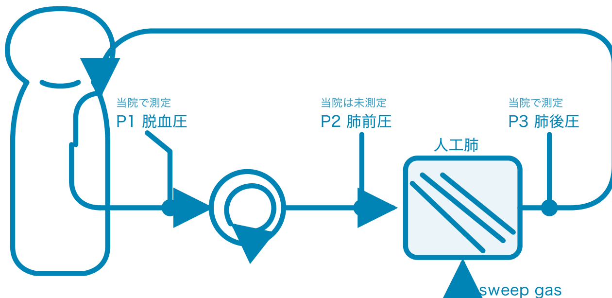
図1. VV-ECMO 回路の全体像と圧の測定点。患者から脱血した血液が遠心ポンプで送られ、人工肺でガス交換されて患者に戻る。P1=脱血圧（ポンプ前・陰圧）／P2=肺前圧（ポンプ後・人工肺前）／P3=肺後圧（人工肺後）。sweep gas は人工肺の気相側に入る。基準値（P1 > -120（当院の運用閾値は -100）／P2 < 300／P2-P3 < 50 mmHg）は §9-1。 当院が測っているのは脱血圧と肺後圧の2点で、肺前圧を測っていないため P2-P3 は算出できない。 モニタ上の番号は図と一部だけ対応する（脱血圧は同じ P1、肺後圧は当院のモニタでは P2=図の P3）ので、 対応表は §9-1 を見ること。
