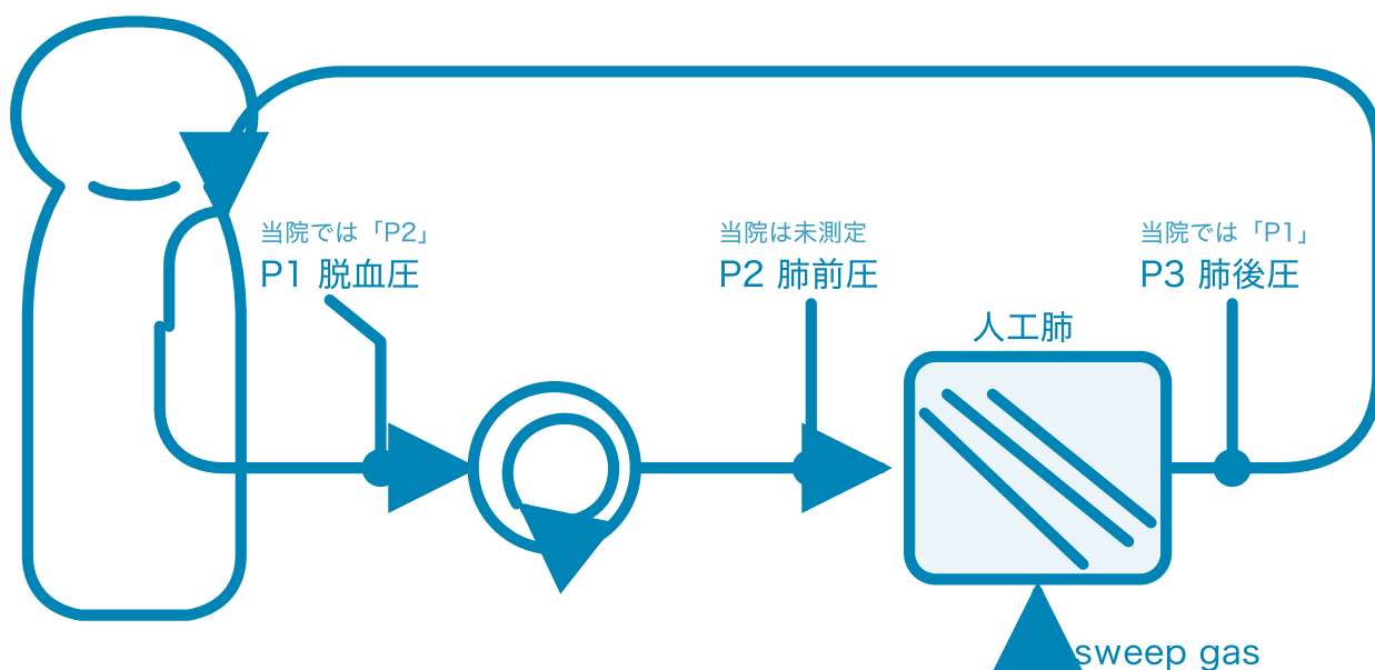
図1. VV-ECMO 回路の全体像と圧の測定点。患者から脱血した血液が遠心ポンプで送られ、人工肺でガス交換されて患者に戻る。P1=脱血圧（ポンプ前・陰圧）／P2=肺前圧（ポンプ後・人工肺前）／P3=肺後圧（人工肺後）。sweep gas は人工肺の気相側に入る。基準値（P1 > -120（当院の運用閾値は -100）／P2 < 300／P2-P3 < 50 mmHg）は §7-1。当院が測っているのは図の P1（脱血圧）と P3（肺後圧）の2点だが、 モニタ上の番号は図と入れ替わっている ——図の P1 が当院の「P2」、図の P3 が当院の「P1」と表示される。肺前圧（図の P2）は測っていないため P2-P3 は算出できない（§7-1）。
