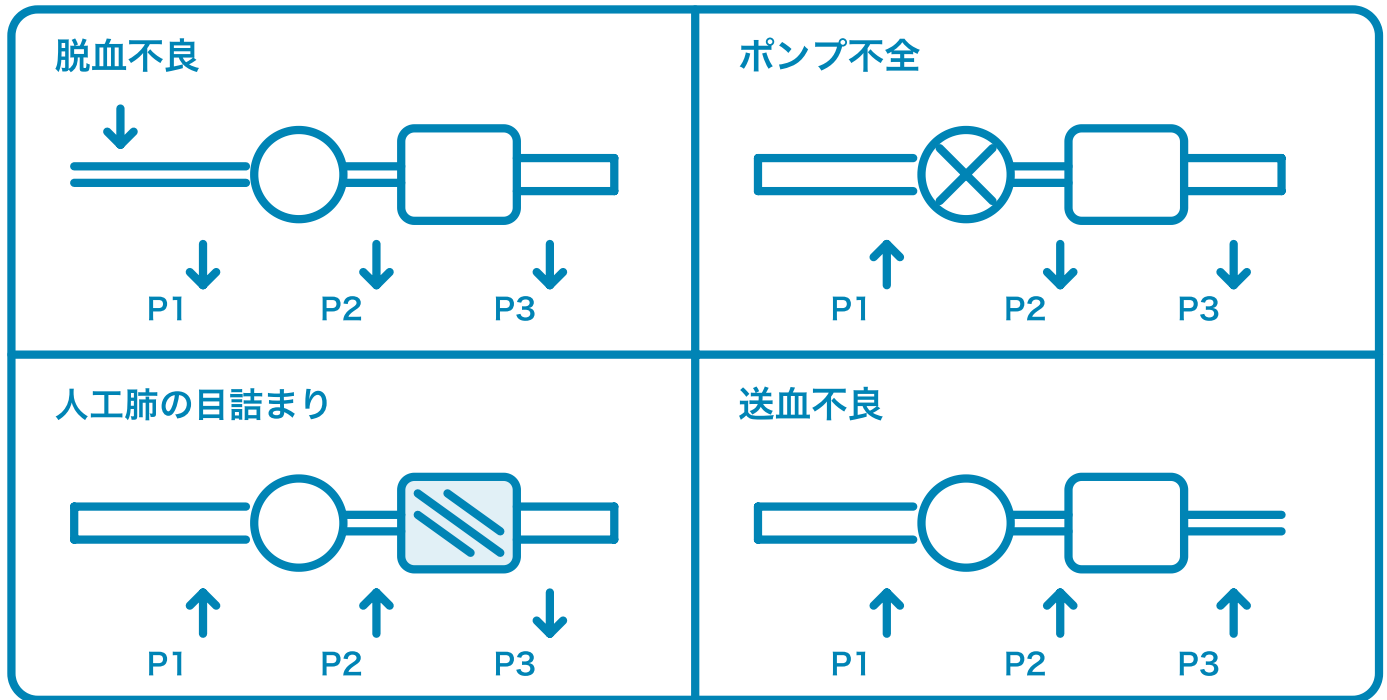
図11. 回路内圧の4象限（表38 の図解）。各象限の下矢印が P1・P2・P3 の動く向き。左上 脱血不良＝P1 が大きな陰圧へ振れ、P2・P3 も下がる（P1 だけが際立って落ちるのが決め手）。右上 ポンプ不全＝P1 が上がり、P2・P3 がともに下がる。左下 人工肺の目詰まり＝P2 が上がり P3 が下がる（P2-P3 が開く）。右下 送血不良＝P2 も P3 も上がる（P2-P3 は開かない）。流量はいずれも低下する。
