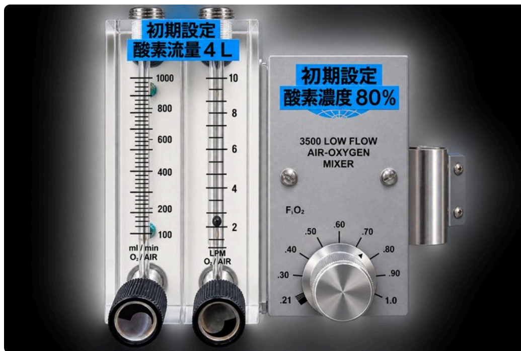
図8. 当院のガスブレンダー（Sechrist 3500 LOW FLOW）。右のダイヤルが FDO 2 、中央の LPM 流量計が sweep gas。左の ml/min 微量計は基本触らない。
