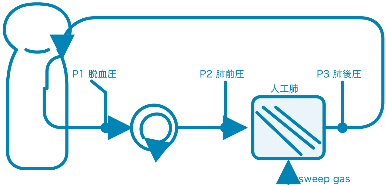
図1. VV-ECMO 回路の全体像と圧の測定点。患者から脱血した血液が遠心ポンプで送られ、人工肺でガス交換されて患者に戻る。P1=脱血圧（ポンプ前・陰圧）／P2=肺前圧（ポンプ後・人工肺前）／P3=肺後圧（人工肺後）。sweep gas は人工肺の気相側に入る。基準値（P1 > -120/P2 < 300/P2-P3 < 50 mmHg）は §7-1。
