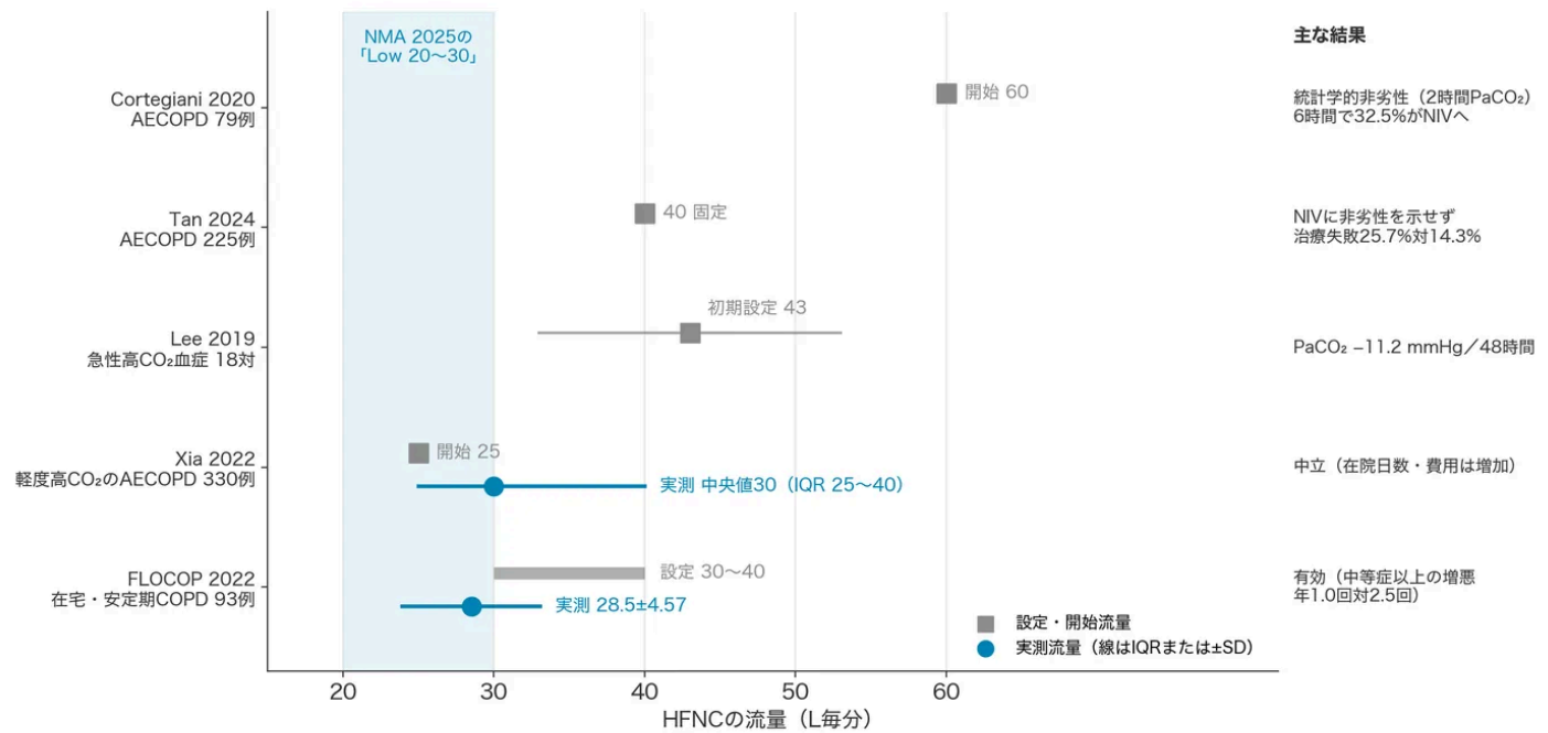
図10. COPDでHFNCを検証した試験の設定流量と実測流量。
