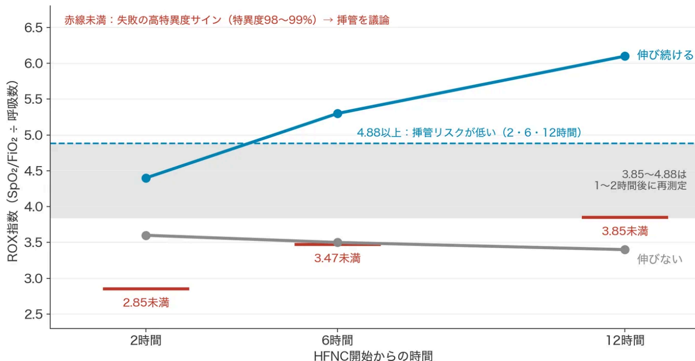
図8. ROX指数の軌道（模式図）と判定の閾値。
