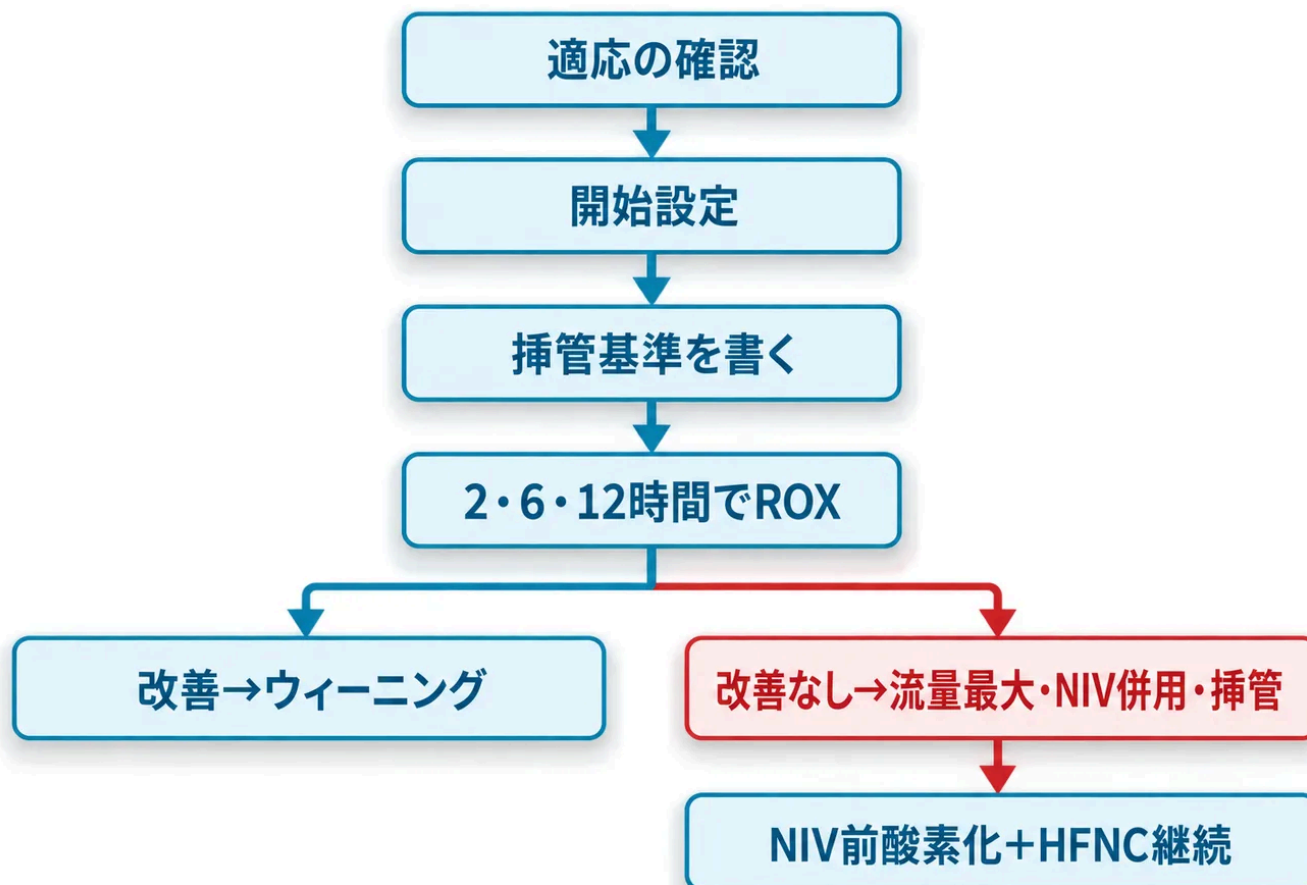
図7. HFNCの流れ — 適応を決め、見切りの基準を書いてから始める。
