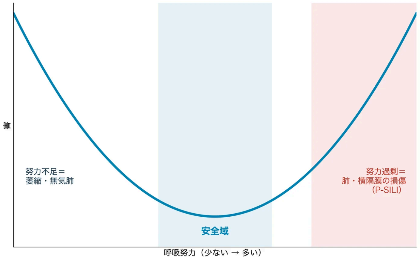
図13. 呼吸努力と害のU字関係。
