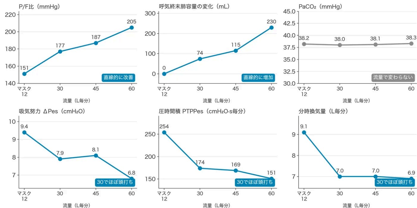
図5. 流量を上げると何が変わるか（非挿管の急性低酸素性呼吸不全17例）。
