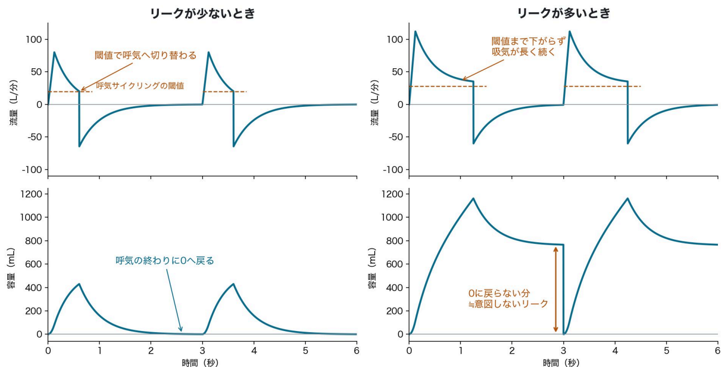
図6. リークが少ないときと多いときの流量と容量の波形（模式図）。
