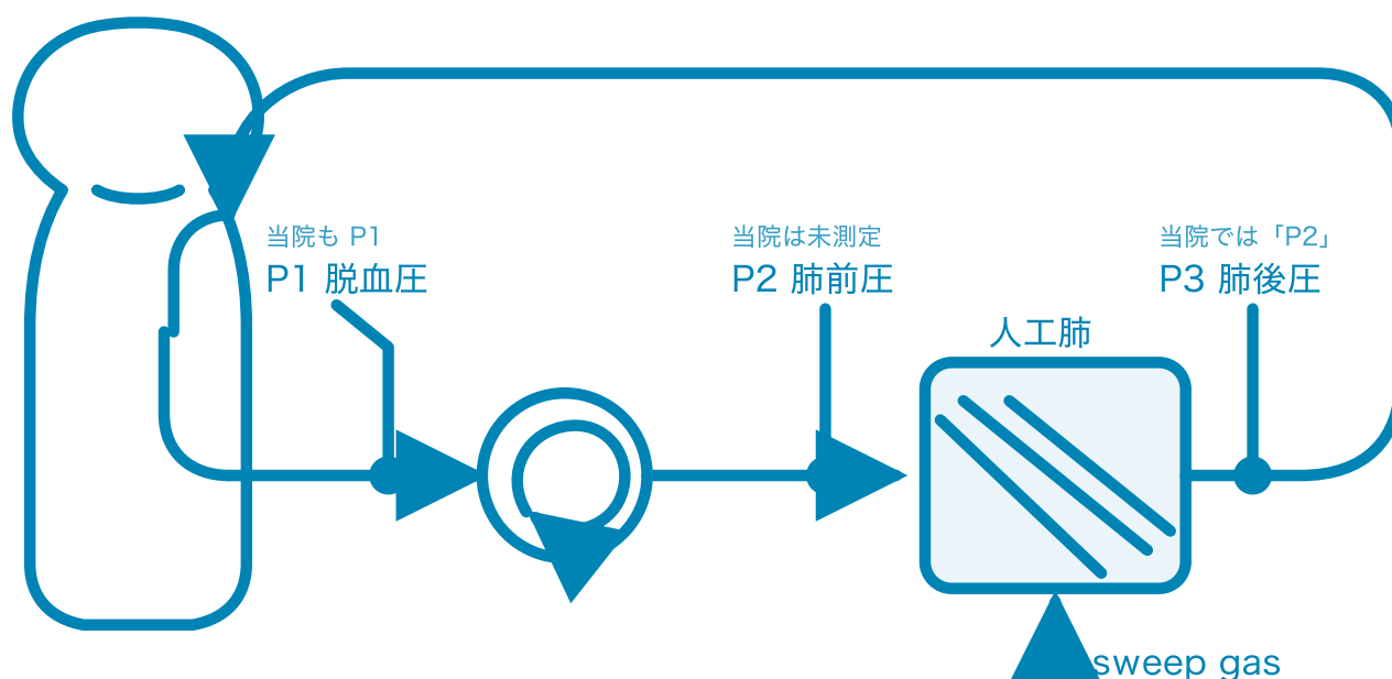
図1. VV-ECMO 回路の全体像と圧の測定点。患者から脱血した血液が遠心ポンプで送られ、人工肺でガス交換されて患者に戻る。P1＝脱血圧（ポンプ前・陰圧）／P2＝肺前圧（ポンプ後・人工肺前）／P3＝肺後圧（人工肺後）。sweep gas は人工肺の気相側に入る。基準値（P1 > -120（当院の運用閾値は -100）／P2 < 300／P2-P3 < 50 mmHg）は §7-1。当院はこの3点のうち P1 と P3 の2点しか測っていない——モニタの「P2」表示は図の P3（肺後圧）で、 肺前圧を測っていないため P2-P3 は算出できない （§7-1）。
