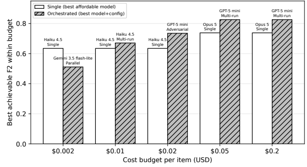
図 2: 項目あたり予算帯ごとに, Single 構成のみで達成可能な最大 F_2 と Orchestrated (Parallel / Adversarial / Multi-run) で達成可能な最大 F_2 を比較. 各棒の上に勝者 (モデル / 構成) を注記. $0.002 では集約コストが吸えず Single が優位, $0.01 で逆転, $0.05 以上では Opus 5 単発すら GPT-5 mini / Multi-run に敗北. $0.05 以上は勝者不変 (予算を 4 倍積んでも改善なし).
