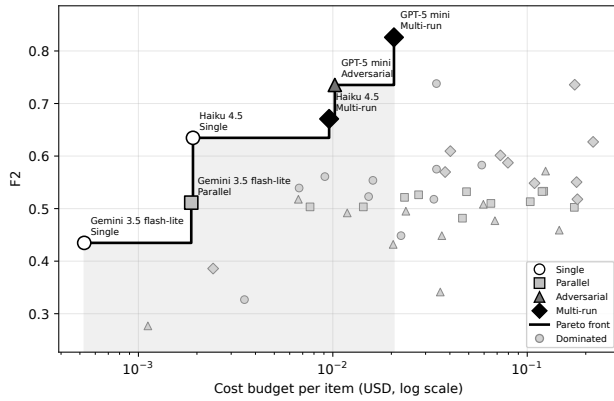
図 1: 項目あたりコスト (対数軸) と F_2 の散布。マーカー形が構成. Pareto 前線 6 点は黒縁で強調しモデル名を注記 (表 2 の P セルに対応), 前線から外れた 42 点はグレー. 前線下のグレー領域は Pareto 支配下.
