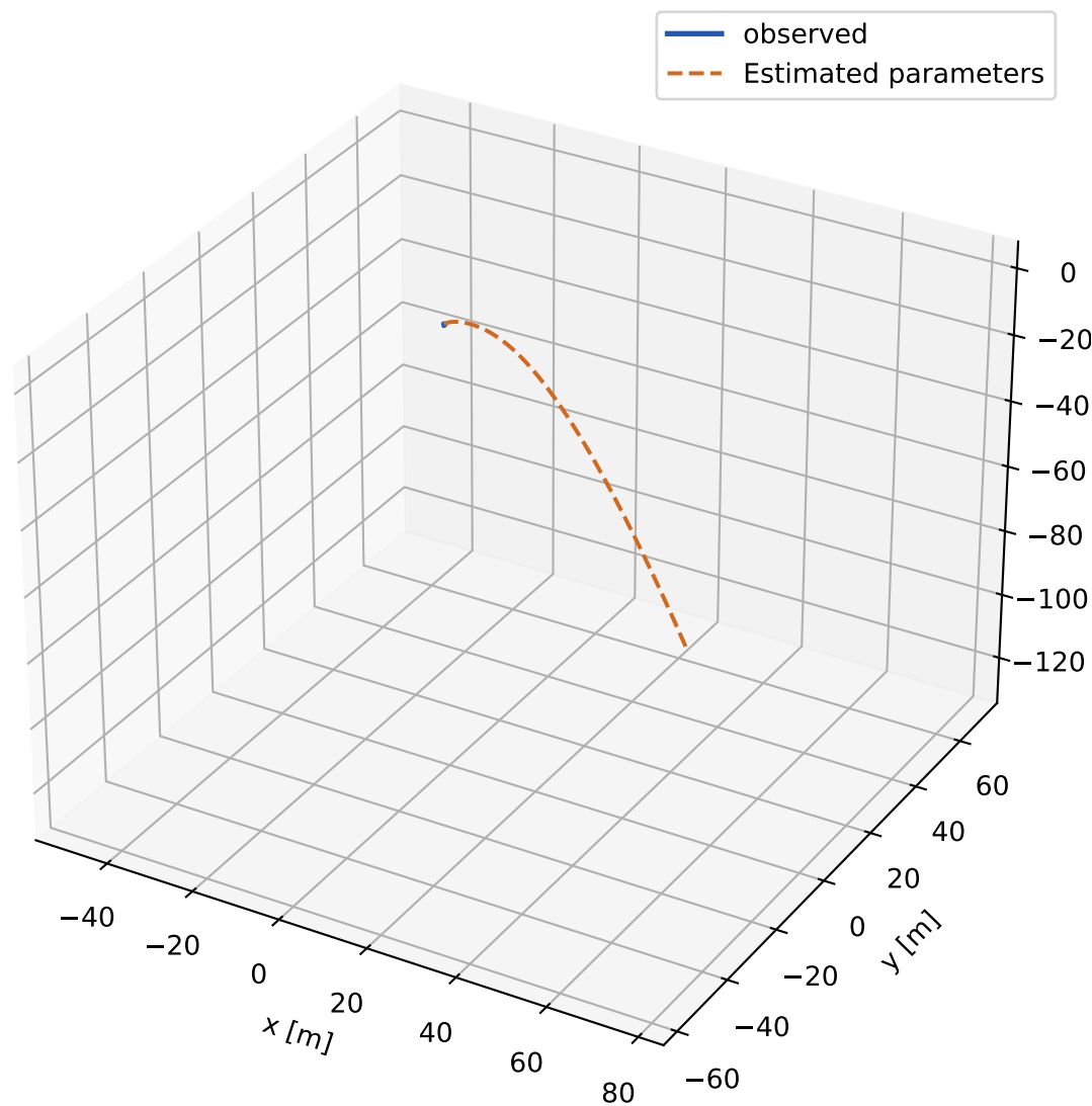
Estimated parameters
