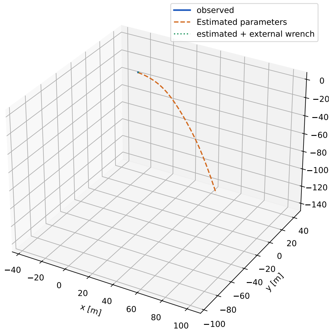
Estimated parameters
