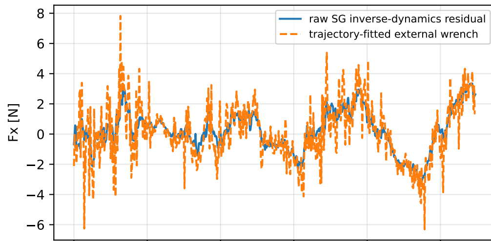
kkt_on_scale_zero: residual wrench
