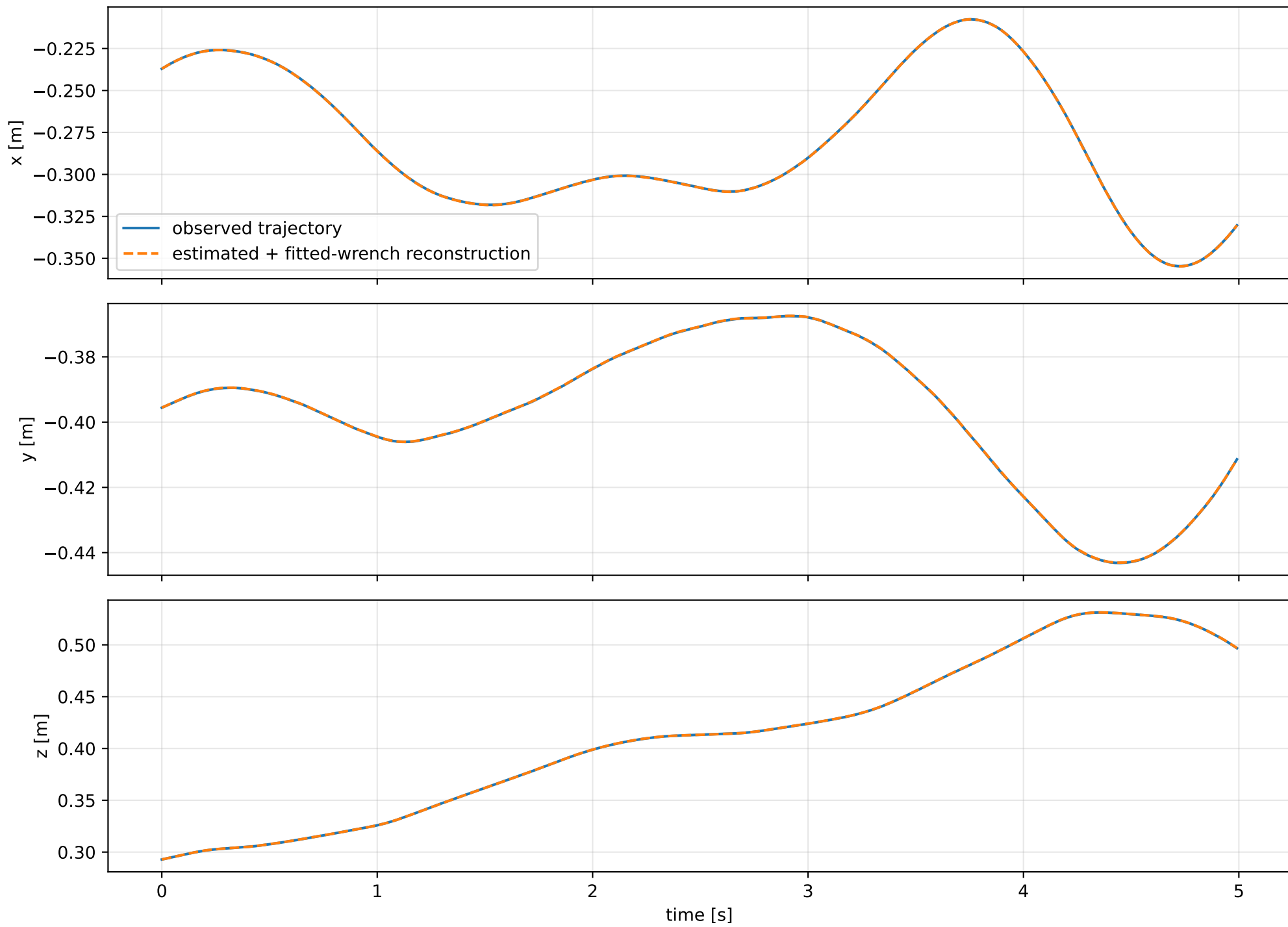
lag_zero: trajectory
