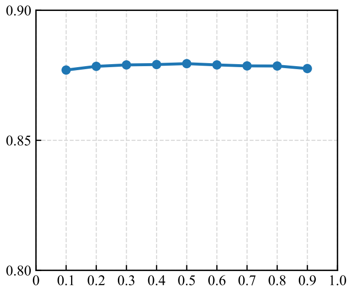
BPIC20RP
