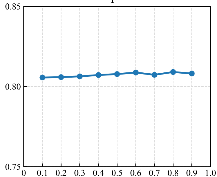
Helpdesk
