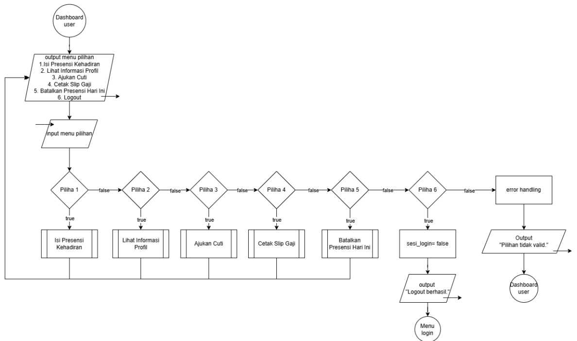
Gambar 2.11 Flowchart Login Sebagai User/Pegawai
