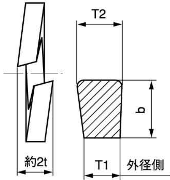
断面A-A
