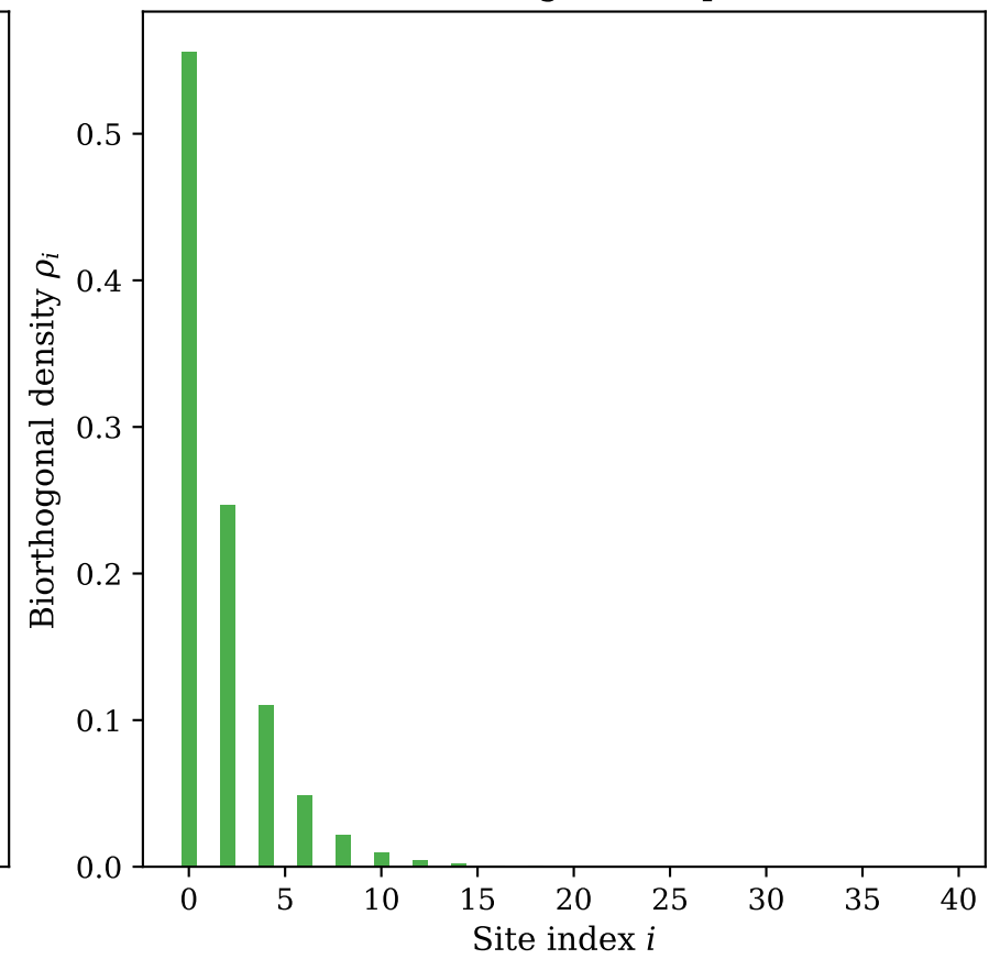
Protected edge mode profile
