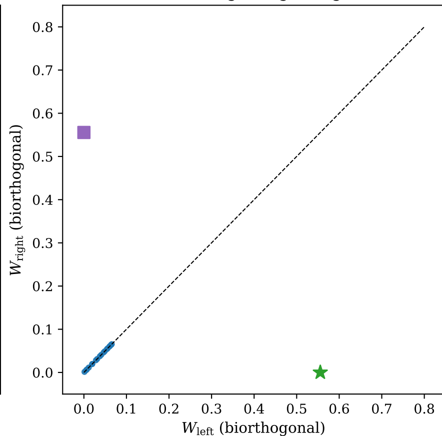
Left vs. right edge weight
