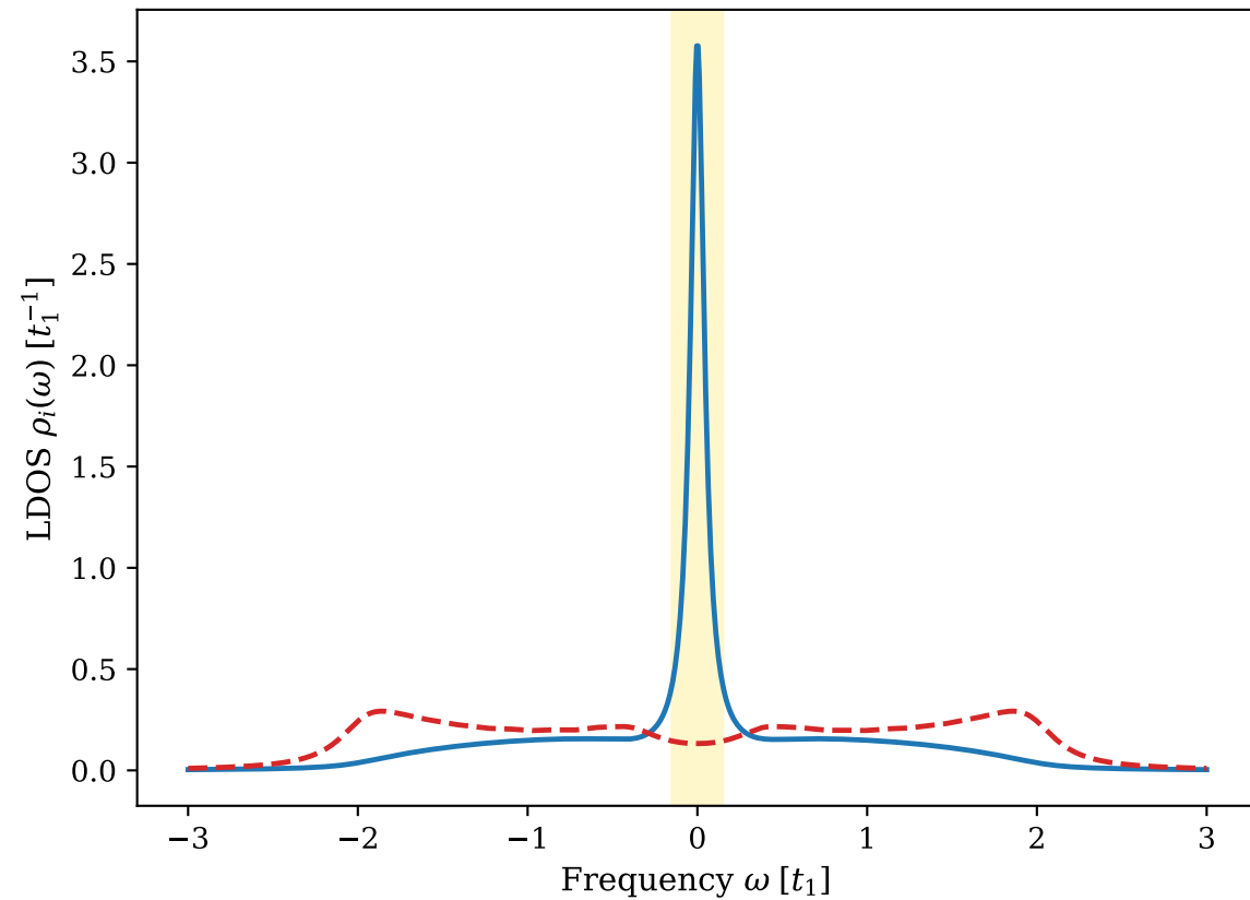
Edge vs. Bulk LDOS
