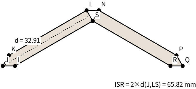
葉A | 上下60°剣先 差し込み部材
