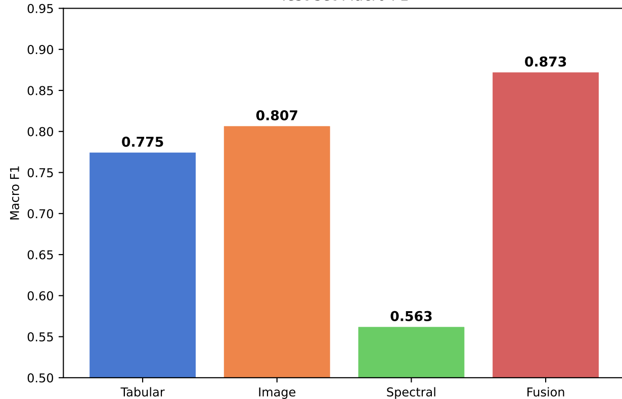
Test-set Macro F1
